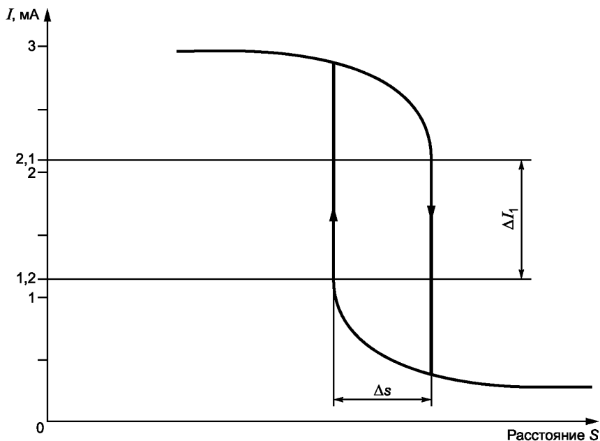
Рисунок 2 — Пример периодической характеристики бесконтактного датчика
