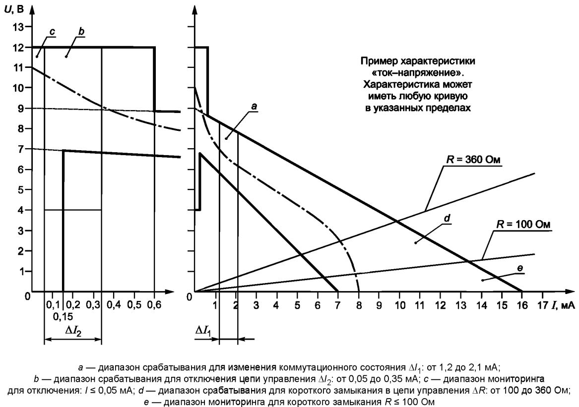
Рисунок 3 — Управляющий ввод коммутирующего усилителя
