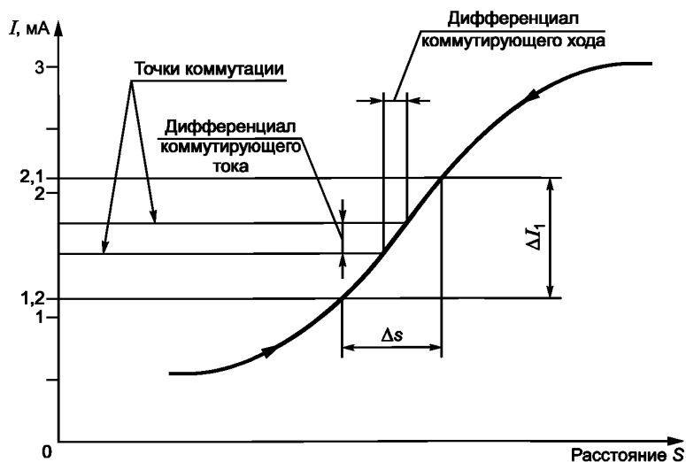
Рисунок 1 — Пример постоянной характеристики бесконтактного датчика
