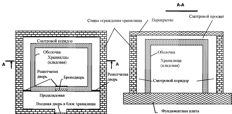
Рисунок 1 – Схематическое устройство хранилища ценностей
