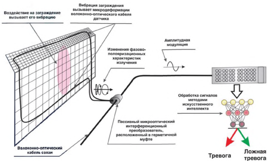
Рисунок 2.45 – Принцип работы системы «Ворон»
