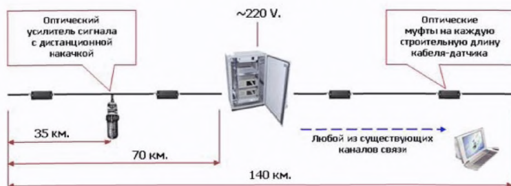
Рисунок 2.47 – Схема одиночного модуля «САМПО»
