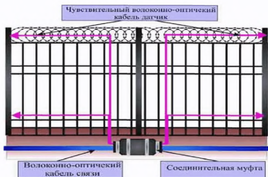
Рисунок 2.46 – Вариант монтажа системы «Ворон»
