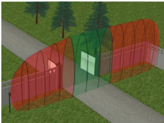
Рисунок 2.5 – 30 извещателя с разделением на подзоны
