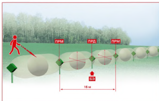
Рисунок 2.11 – ЗО извещателя «Наст»
