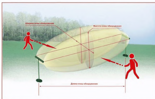
Рисунок 2.10 – ЗО извещателя «Торос»
