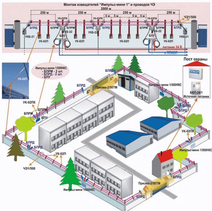
Рисунок 2.16 – Вариант защиты периметра с применением извещателя «Импульс-мини»
