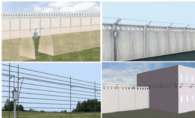
Рисунок 2.14 – Варианты установки проводноволнового извещателя
