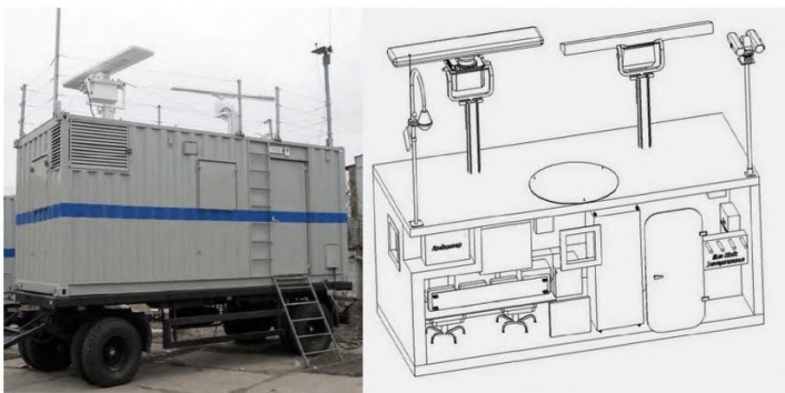
Рисунок 2.56 – Внешний вид «НЕВА-МП» в комплексе со средствами электрооптического обнаружения
