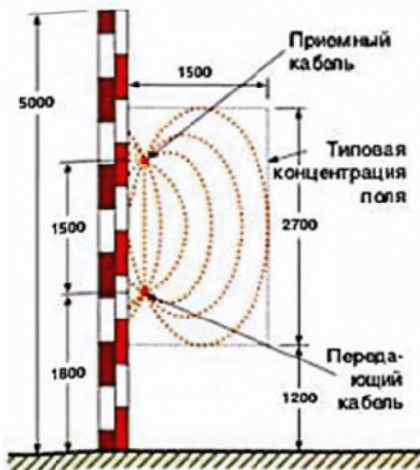
Рисунок 2.19 – Типовая ЗО при установке ЧЭ на стене
