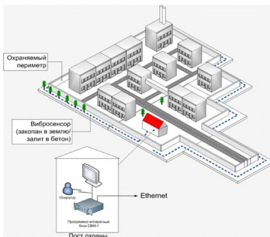
Рисунок 2.49 – Применение ВОС охраны периметра «СВМ-1»
