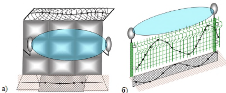
Рисунок 2.51 – Примеры охраны ограждений извещателем «Рубеж»
