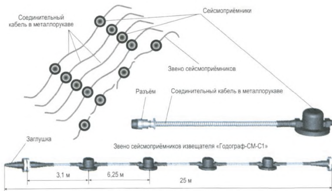
Рисунок 2.29 – ЧЭ сейсмического извещателя «Годограф-СМ-С-1»
