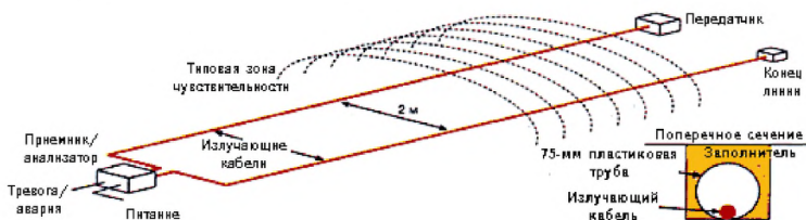
Рисунок 2.17 – Структурная схема ЛВВ-извещателя
