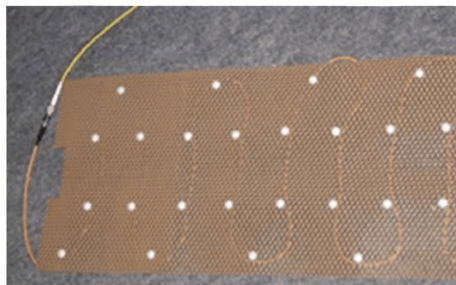
Рисунок 2.25 – Установка кабеля на сетке
