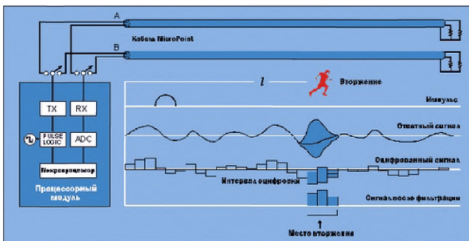
Рисунок 2.44 – Процесс обнаружения нарушителя
