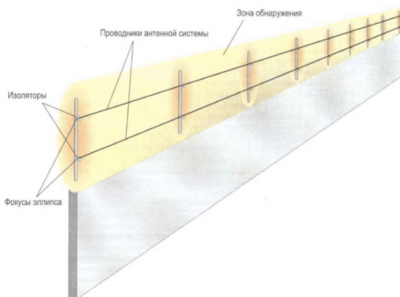
Рисунок 2.1 – ЗО емкостного извещателя
