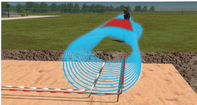
Рисунок 2.18 – Типовая ЗО при установке ЧЭ в грунт
