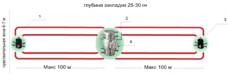
Рисунок 2.33 – Четырехтрубная версия
