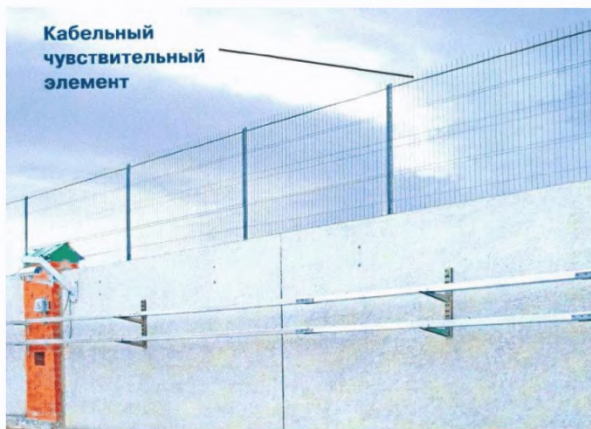
Рисунок 2.38 – Установка вибрационного извещателя
