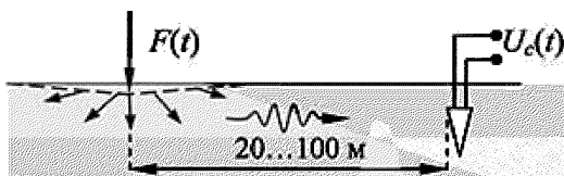
Рисунок 2.22 – Взаимодействие объекта обнаружения через грунт с ЧЭ
