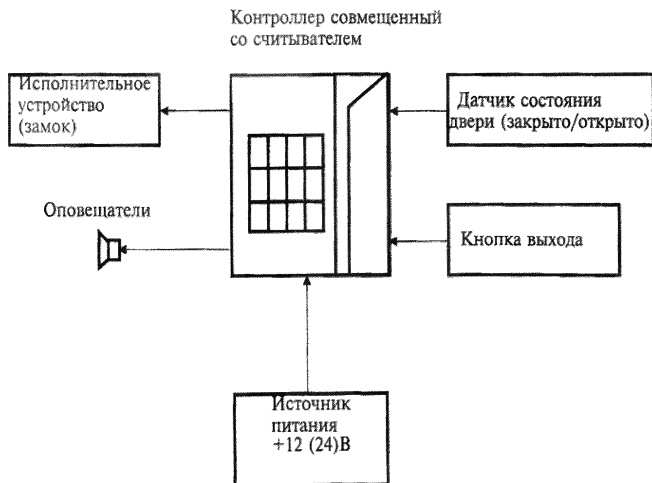
Рисунок 1 – Оборудование СКУД помещения с одной дверью
