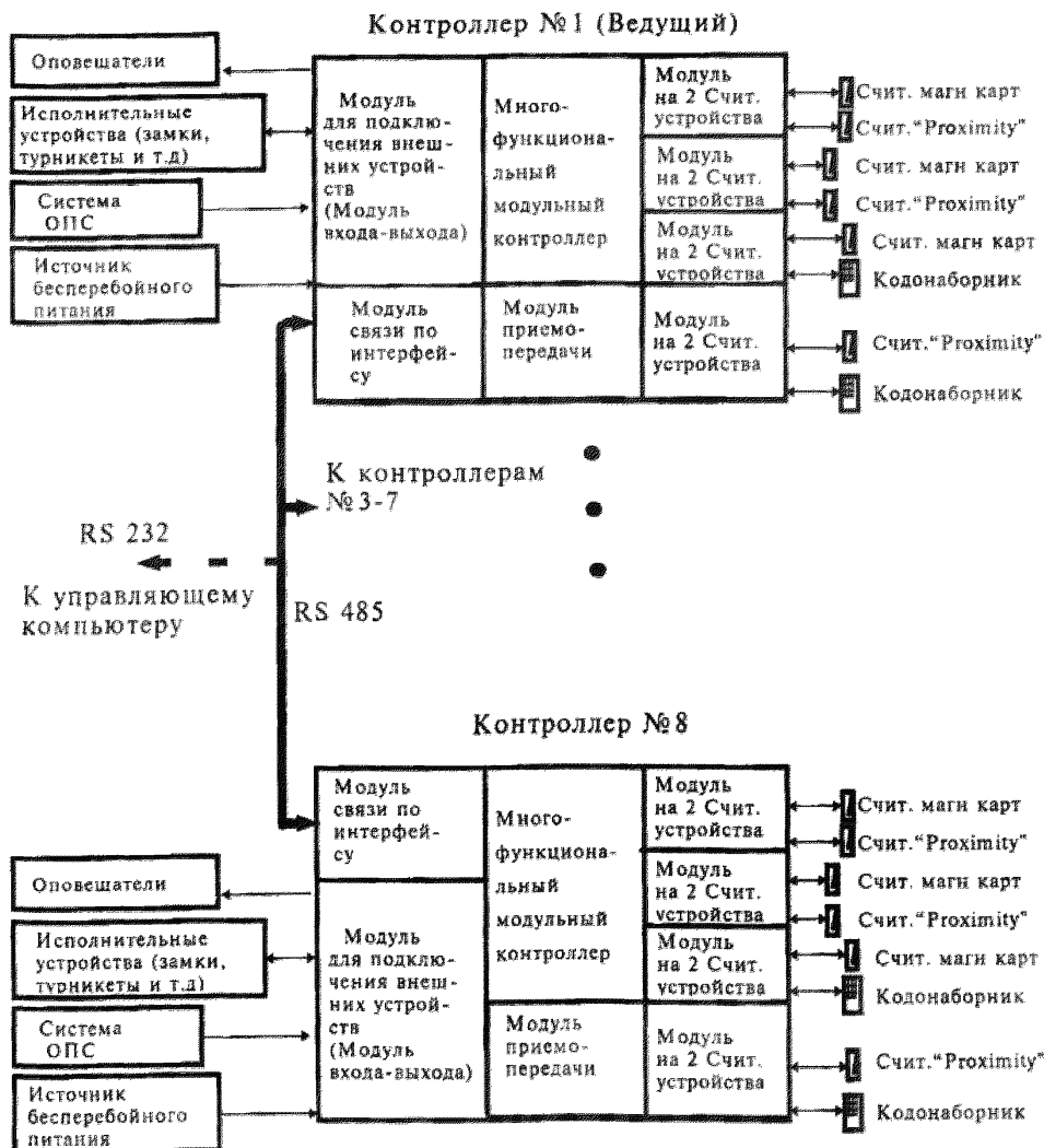
Рисунок 3 – Примерная структурная схема построения сетевой СКУД
