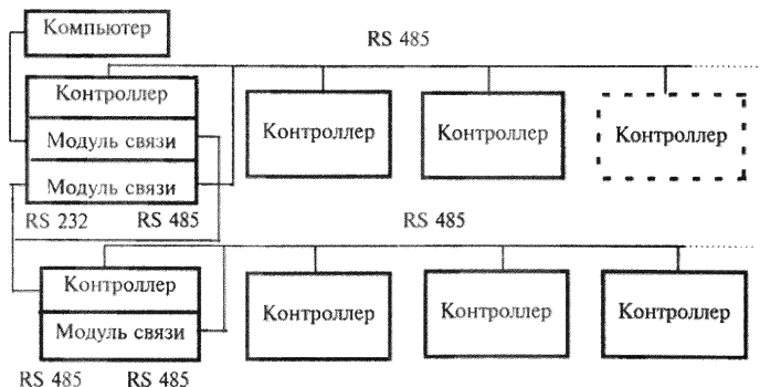
Рисунок 5 – Примерная структурная схема построения сетевой СКУД с несколькими ветвями
