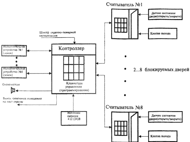
Рисунок 2 – Оборудование СКУД объекта с несколькими дверьми
