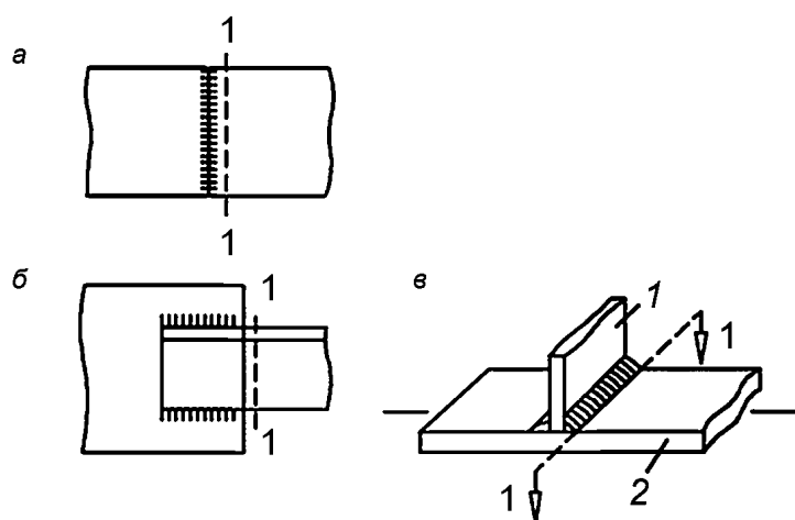
а — встык; б — внахлестку фланговыми швами; в — схема прикрепления поперечного элемента 1 к элементу 2, не имеющему стыка; 1-1 — расчетное сечение
