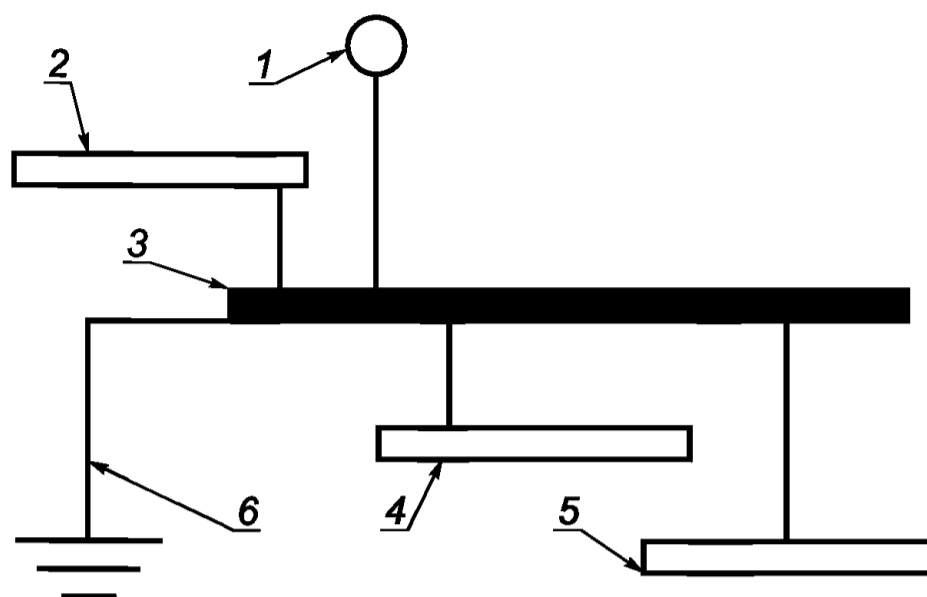
1 — антистатический браслет (манжета и шнур заземления); 2 — рабочая поверхность; 3 — общая точка заземления; 4 — напольное антистатическое покрытие; 5 — антистатический пол; 6 — функциональное заземление или защитное заземление (функциональное заземление должно соединяться с защитным заземлением)
