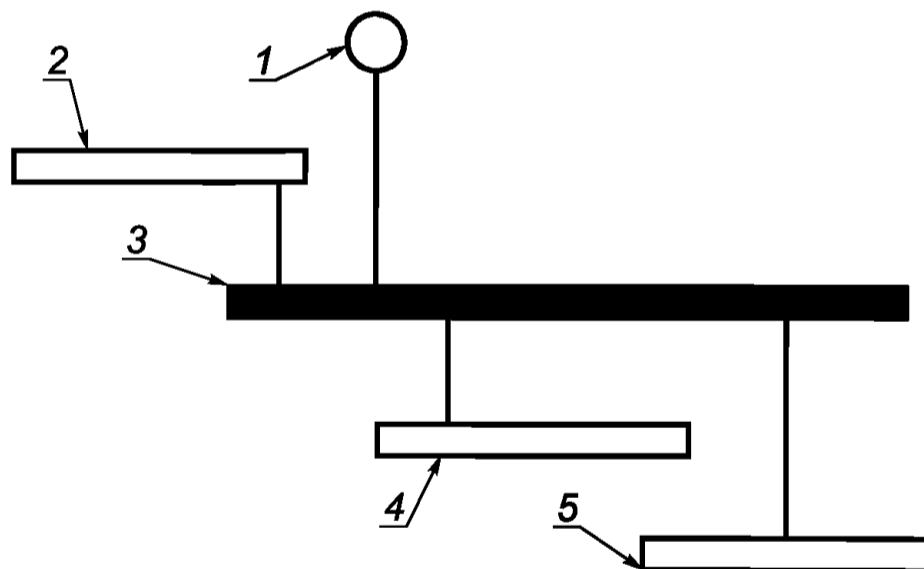
1 — антистатический браслет и шнур; 2 — рабочая поверхность; 3 — общая точка заземления; 4 — напольное антистатическое покрытие; 5 — антистатический пол
