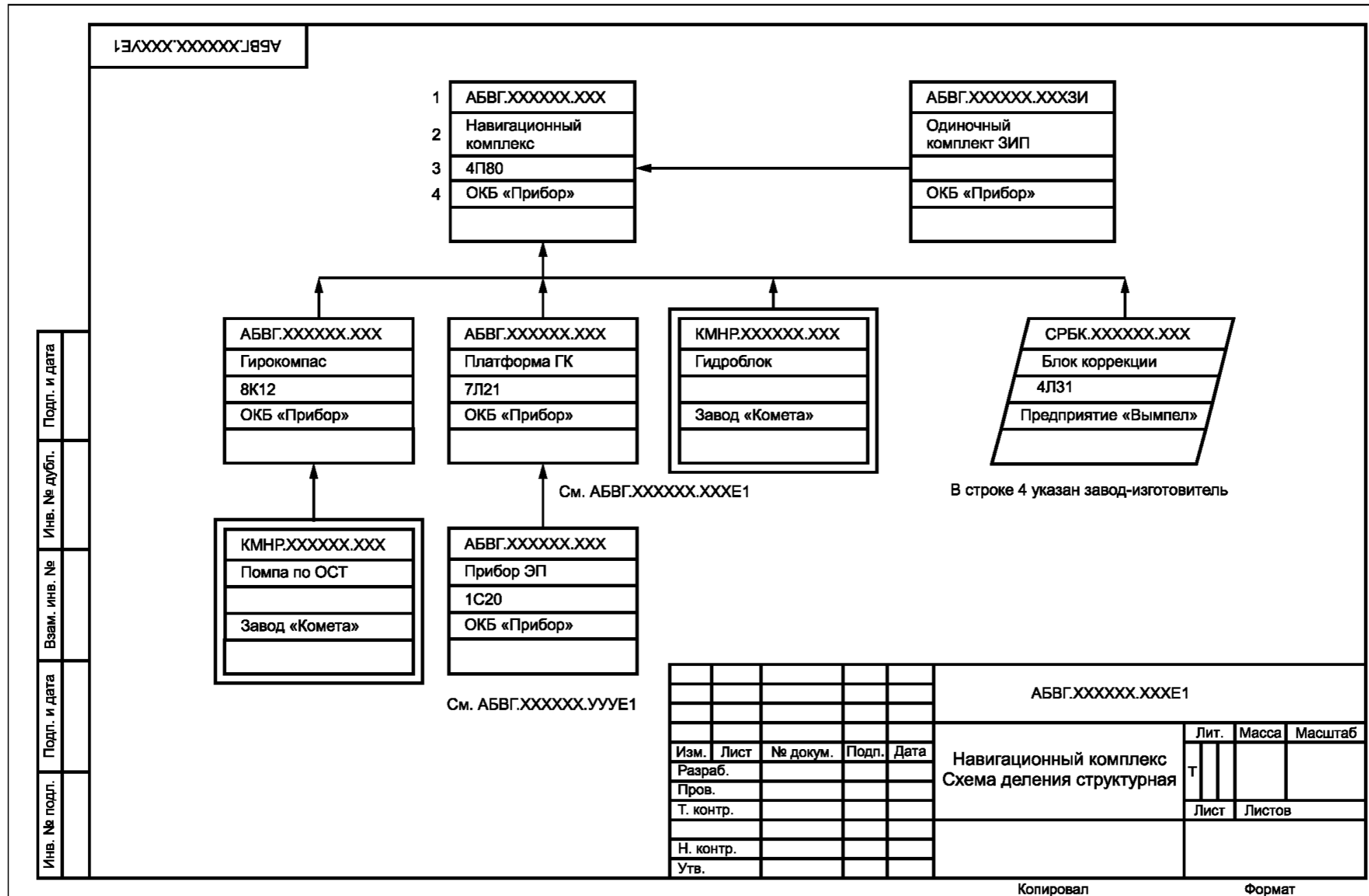
Рисунок Б.1 — Пример оформления схемы деления изделия при выполнении в бумажной форме
