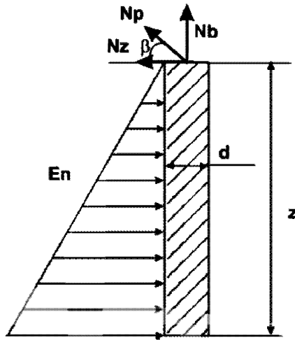
Рисунок Е.1 – Общая схема к расчёту анкеров
