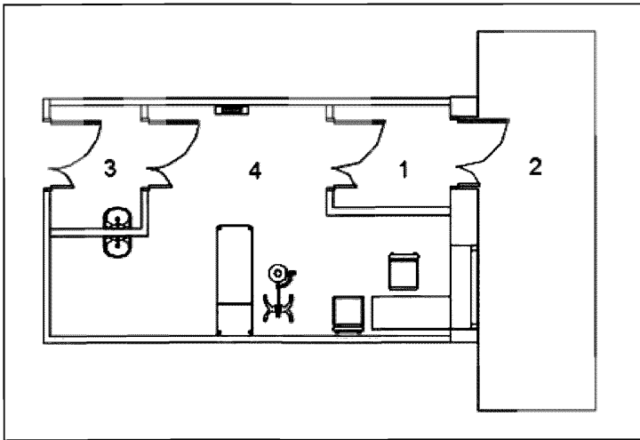
Рисунок 14 – Планировочное решение приемно-смотрового бокса: 1 – наружный тамбур; 2 – открытая галерея; 3 – шлюз для персонала; 4 – смотровая
