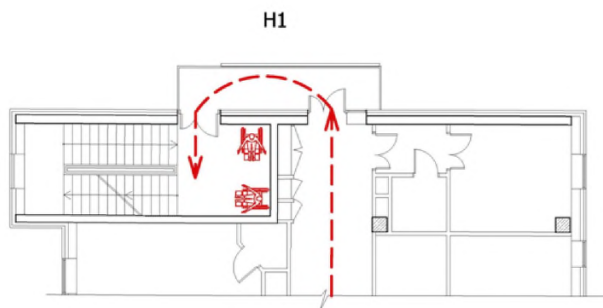
Рисунок 101 – Пример проектного решения незадымляемой лестничной клетки N1
