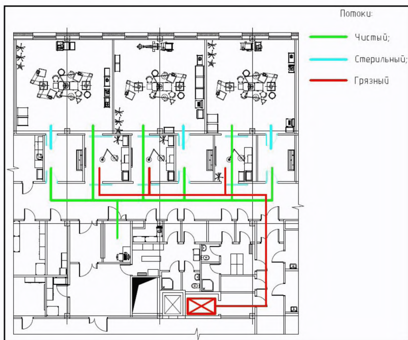
Рисунок 31 – Пример планировочного решения операционного блока на 3 операционных
