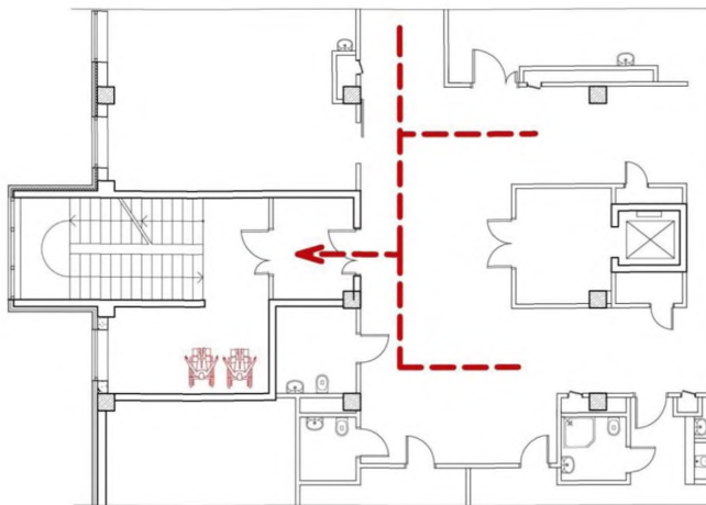
Рисунок 102 – Примеры проектных решений незадымляемых лестничных клеток Н2, Н3
