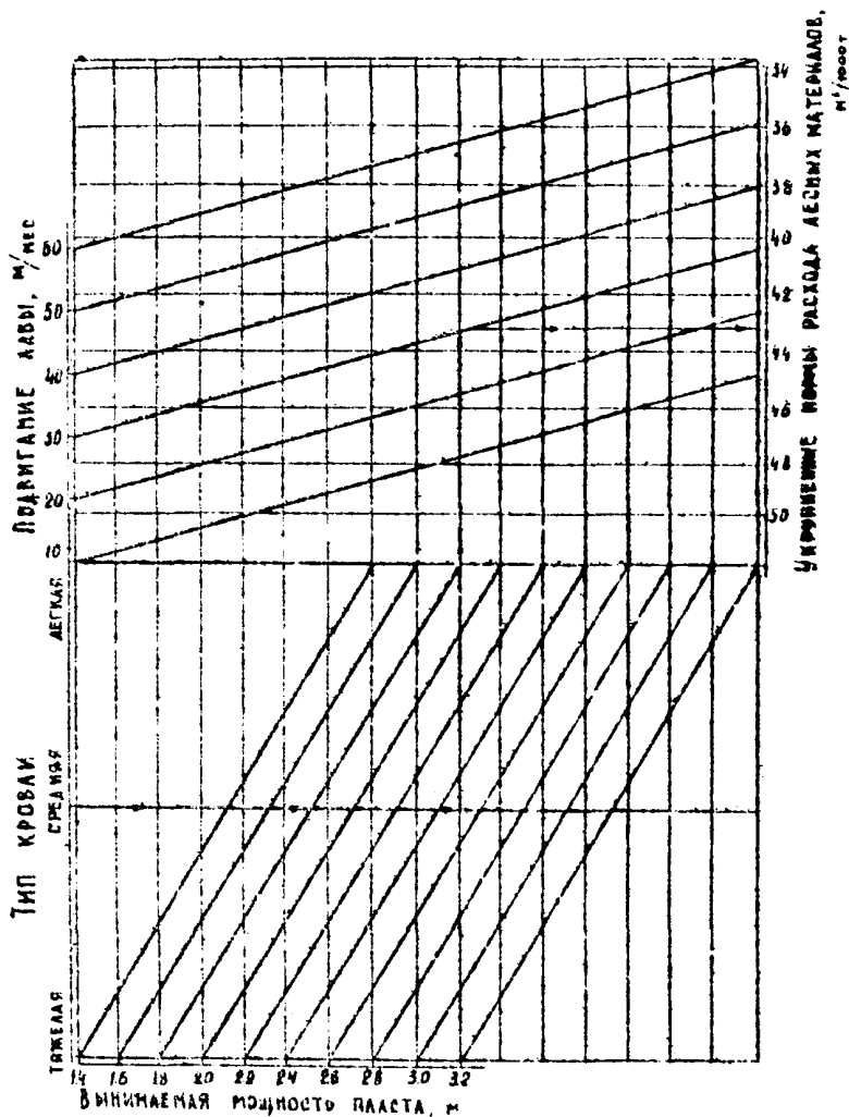
Рис. 4. Номограмма для определения укрупнения норм расхода лесных материалов на кровле очистных выработок.
