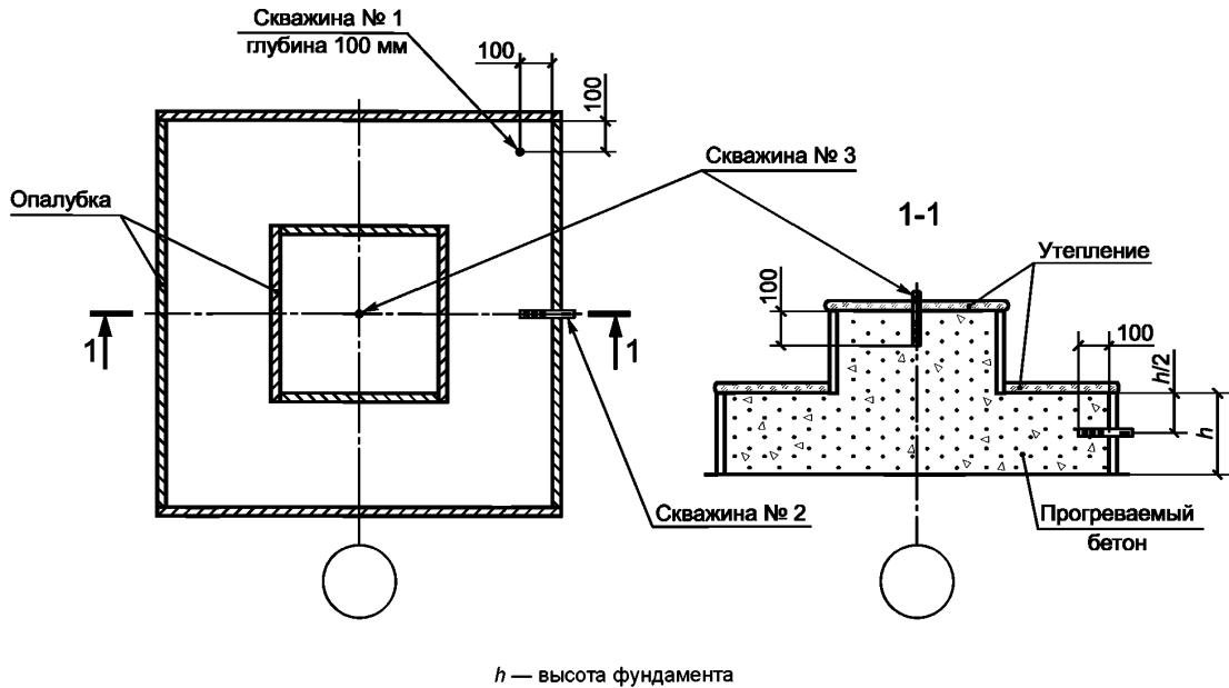
Рисунок 10.6 — Схема расстановки температурных скважин в отдельном фундаменте
