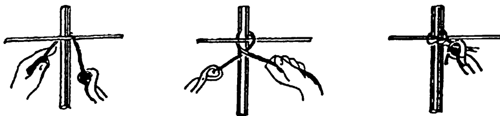
Рисунок 7.1 — Вязка узлов без подтягивания
