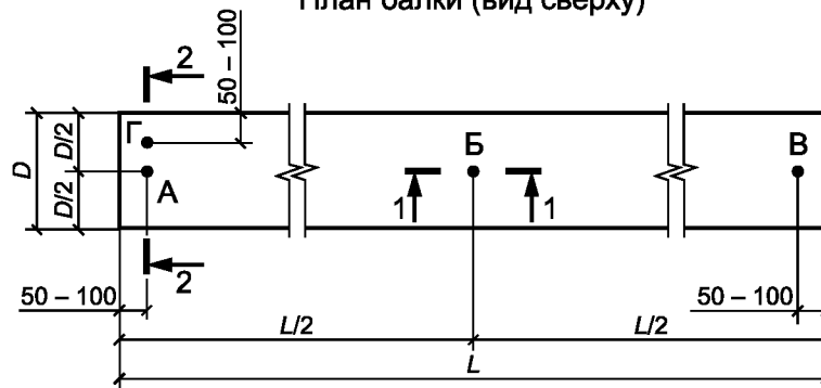
План балки (вид сверху)
