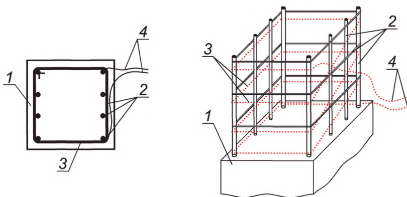
1 — фундамент; 2 — арматура; 3 — греющий провод; 4 — выпуски греющего провода для подключения к питающим электрическим проводам (места подключения должны находиться в бетоне)
