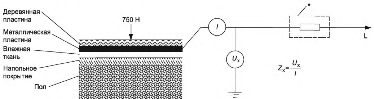
Рисунок В.2 — Испытательный электрод 2
