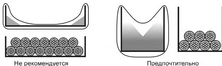
Рисунок 44.R19 — Прокладка кабелей в металлических кабельных лотках
