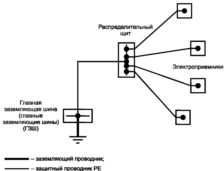
Рисунок 44.R13 — Пример радиального соединения защитных проводников РЕ
