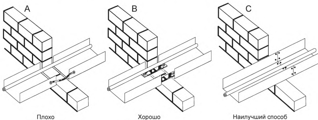
Рисунок 44.R22 — Соединение металлических секций
