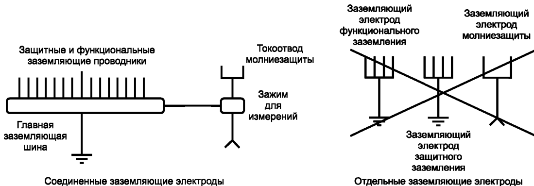
Рисунок 44.R12 — Взаимосоединенные заземляющие электроды
