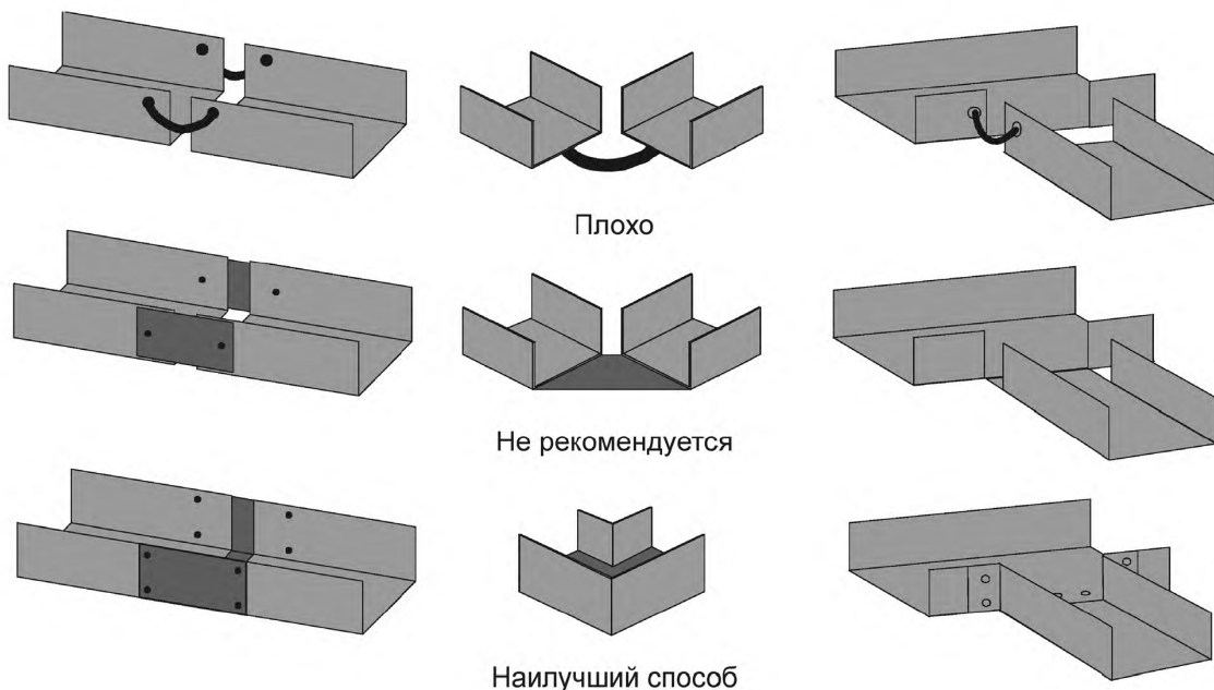
Рисунок 44.R20 — Непрерывность системы, состоящей из металлических элементов
