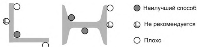
Рисунок 44.R21 — Расположение кабелей внутри элементов металлических конструкций
