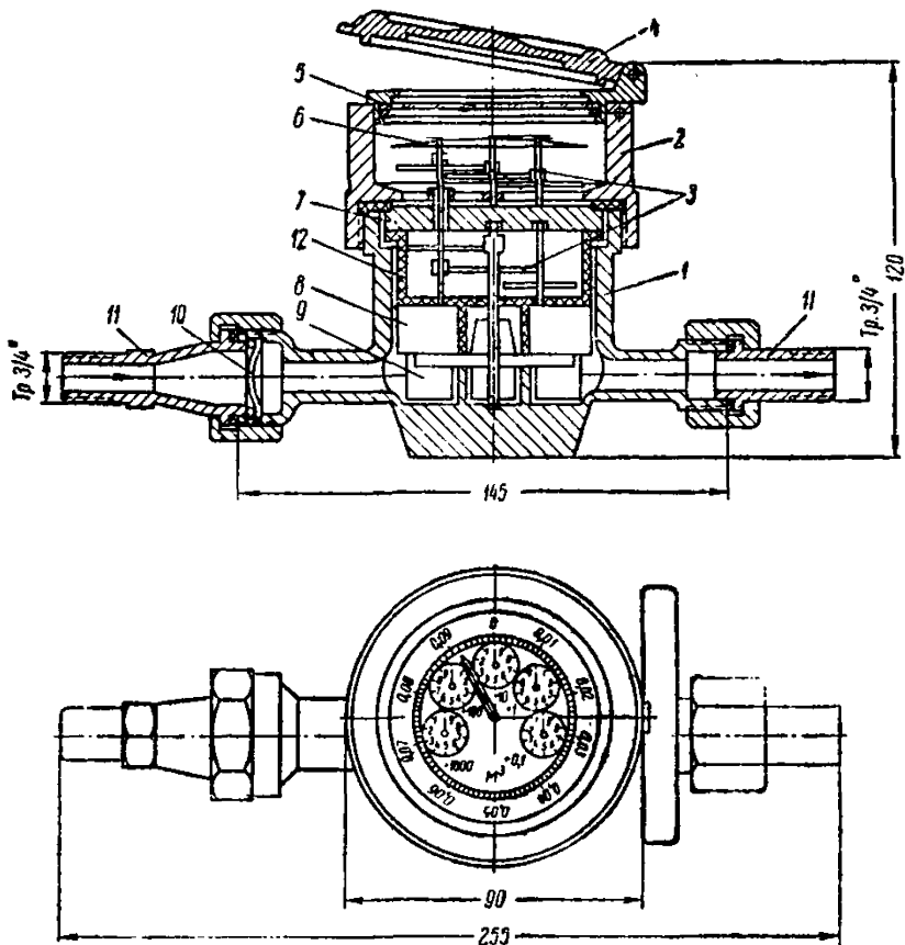
Рис. 32. Водомер типа ВК:
