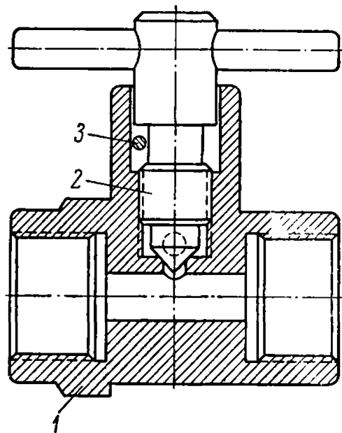
Рис. 27. Вентиль разгрузочный: 1 — корпус; 2 — шток; 3 — кольцо
