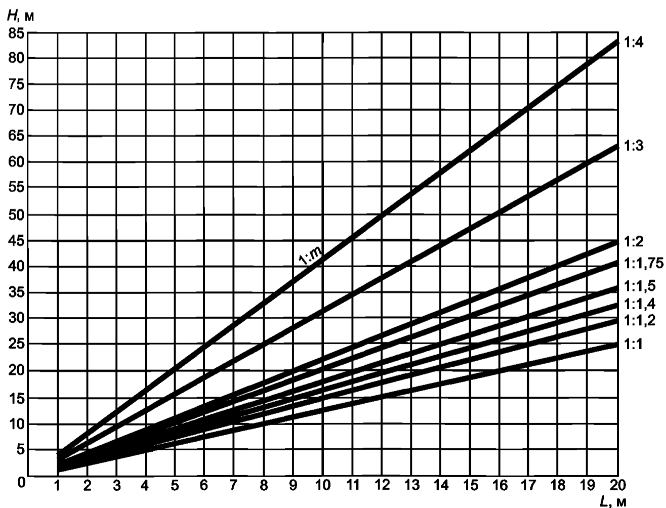
Рисунок 8.1 — Определение длины склона (откоса) L в зависимости от высоты H и величины заложения склона (откоса) 1:m
