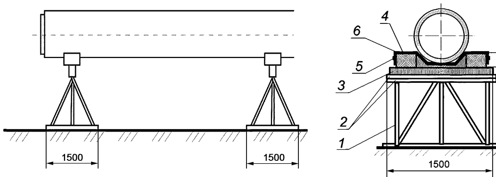
1 — основание (уголок 50 × 50 × 5 мм); 2 — швеллеры № 16; 3 — брус (100 × 150 × 1500 мм); 4 — ложемент (брус 500 × 200 мм); 5 — саморез; 6 — эластичная накладка (резина по ГОСТ 7338) шириной 500 мм и толщиной не менее 20 мм
