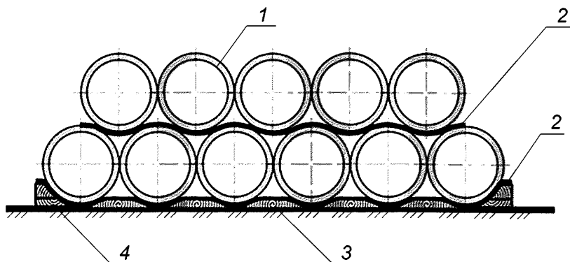
Рисунок 8 — Пример схемы устройства штабеля и крепления теплоизолированных труб
