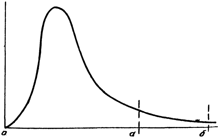
Рис. I. Характерный вид кривой отмывки фильтрующей загрузки
