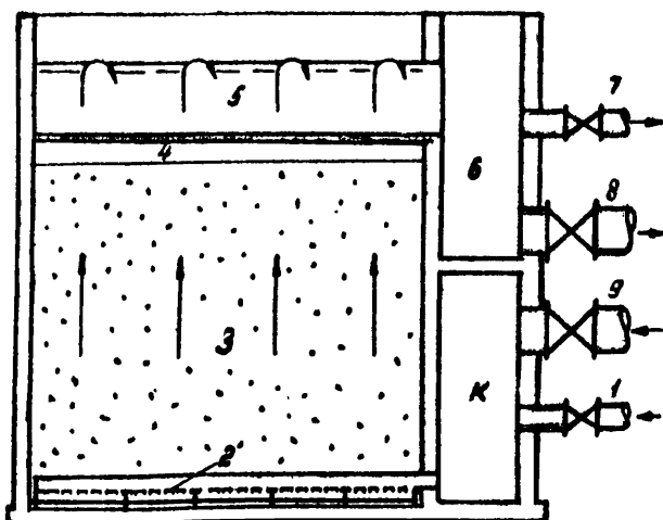
Рис. 1. Схема устройства контактного осветителя типа КО-1 (в безгравийном варианте)
