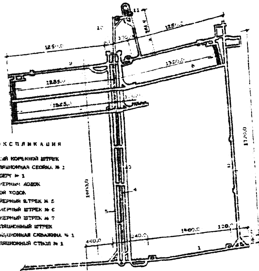
РИС.7.6. ПОДГОТОВКА ПАНЕЛИ №1
