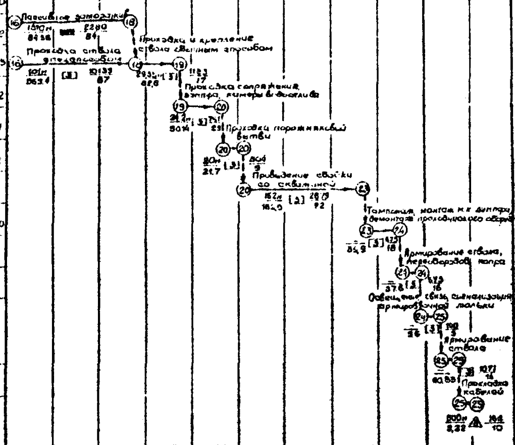
РИС.7 И. ПОДУЗЕЛ 2.2. ПРОХОДКА И АРМИРОВАНИЕ ВЕНТИЛЯЦИОННОГО СТВОЛА №1
