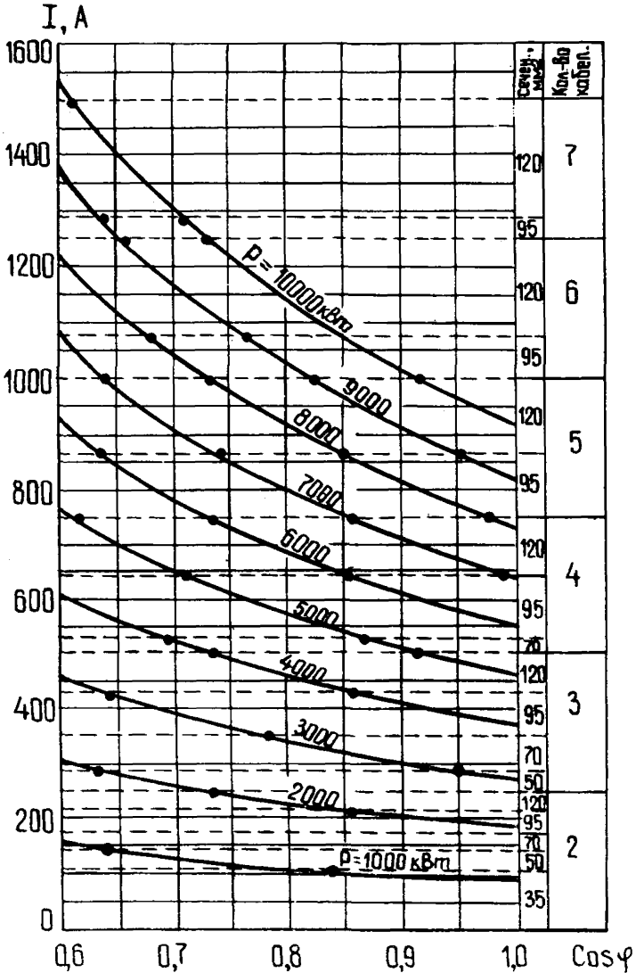
Рис.2.3. Диаграмма определения числа ствольных кабелей и их сечений
