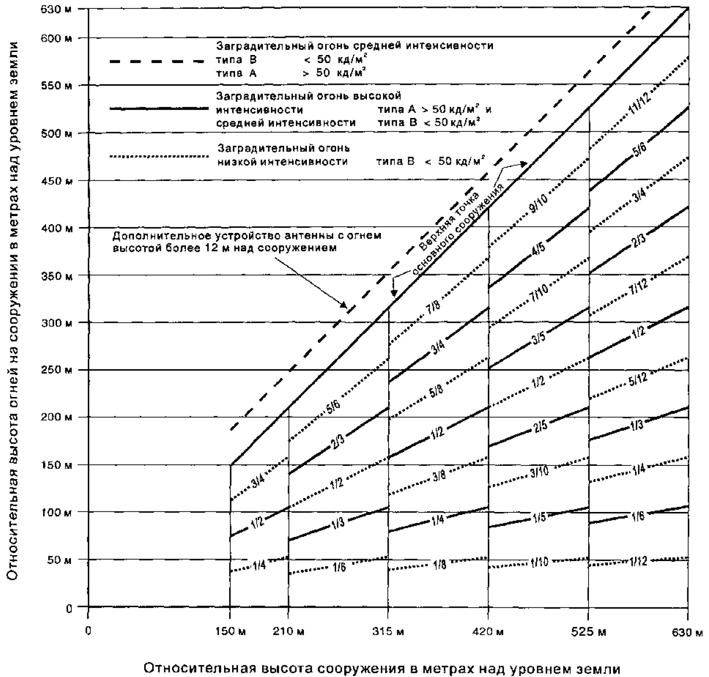
Рис. Д.7.5. Сдвоенная система светозащиты препятствий с огнями высокой/средней интенсивности типа А/типа В
