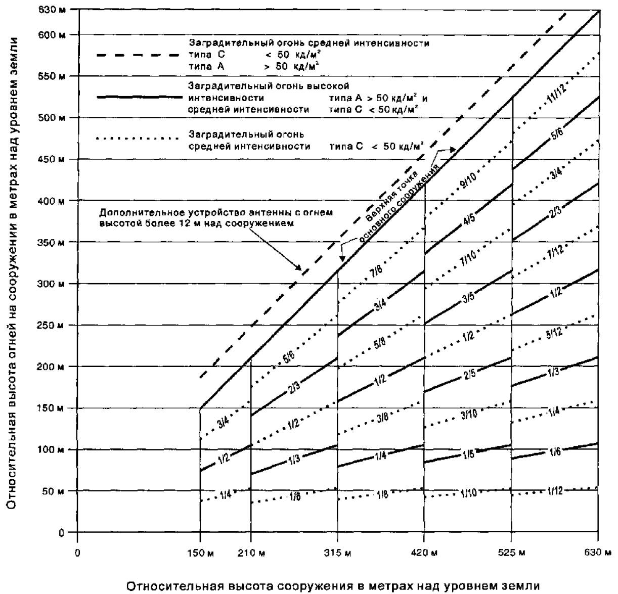
Рис. Д.7.6. Сдвоенная система светоограждения препятствий с огнями высокой/средней интенсивности типа А/типа С
