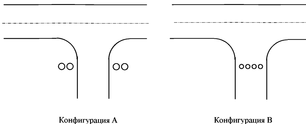
Рис. 5.26. Огни защиты ВПП.
