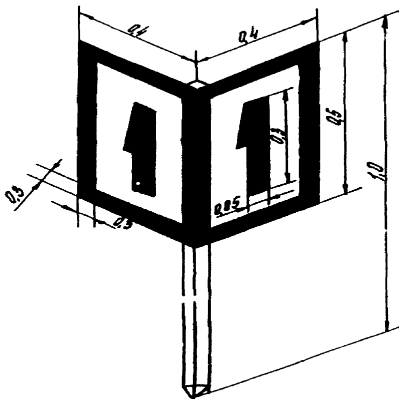
Рис. П.6.6. Знак МС
