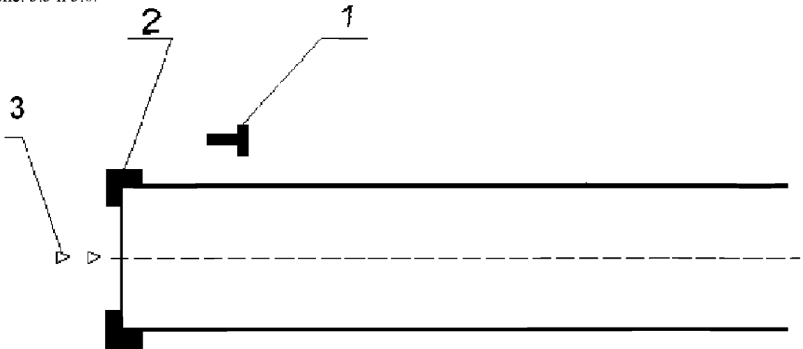
Рис. 5.5. Схема оборудования маркировочными знаками ГВПИ класса А, Б, В, Г, Д: 1 – маркировка посадочного «Т»; 2 – угловой маркировочный знак; 3 – осевой маркировочный знак
