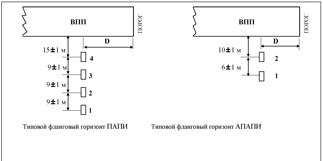
Рис. 5.22. Расположение систем ПАПИ и АПАПИ
