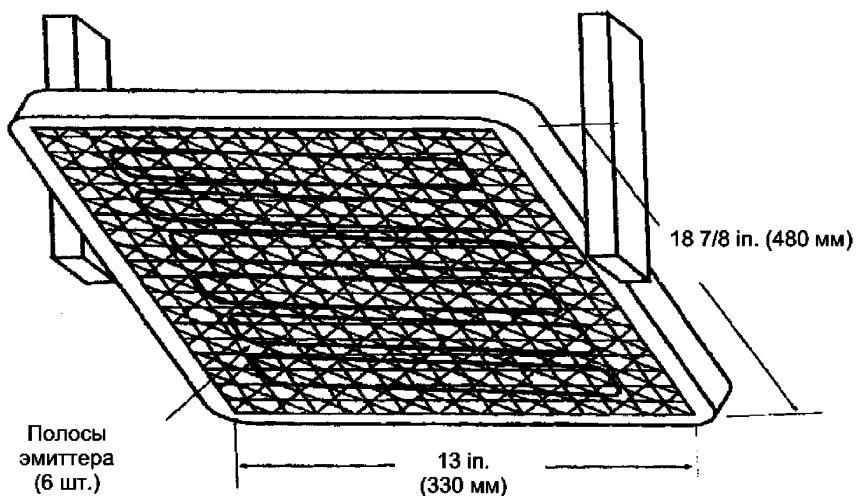
Рис. 3а. Электрическая панель теплового излучения
