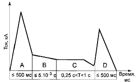
Рис. 1. Форма и параметры тока молнии
