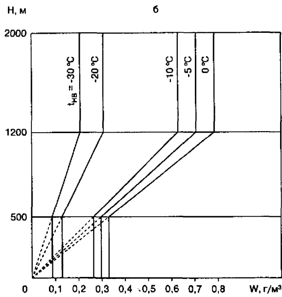
Рис. 2. Зависимость влажности от вертикальной протяженности зоны обледенения а – L = 200 км; б – L = 32 км
