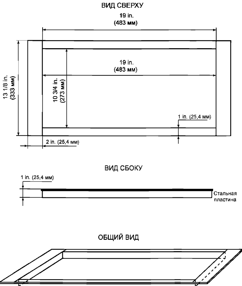
Рис. 5. Крепежная рама
