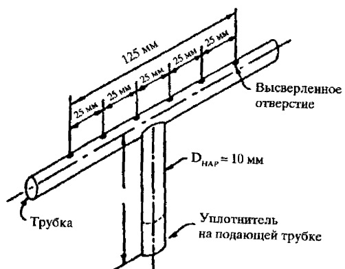
Рис. 4. Горелка
