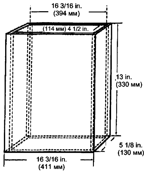
Рис. 2. Вытяжная труба
