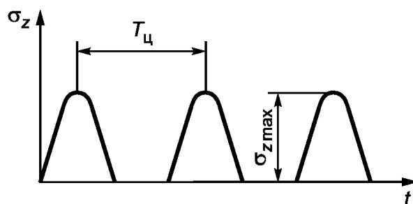
б) цикл напряжений
