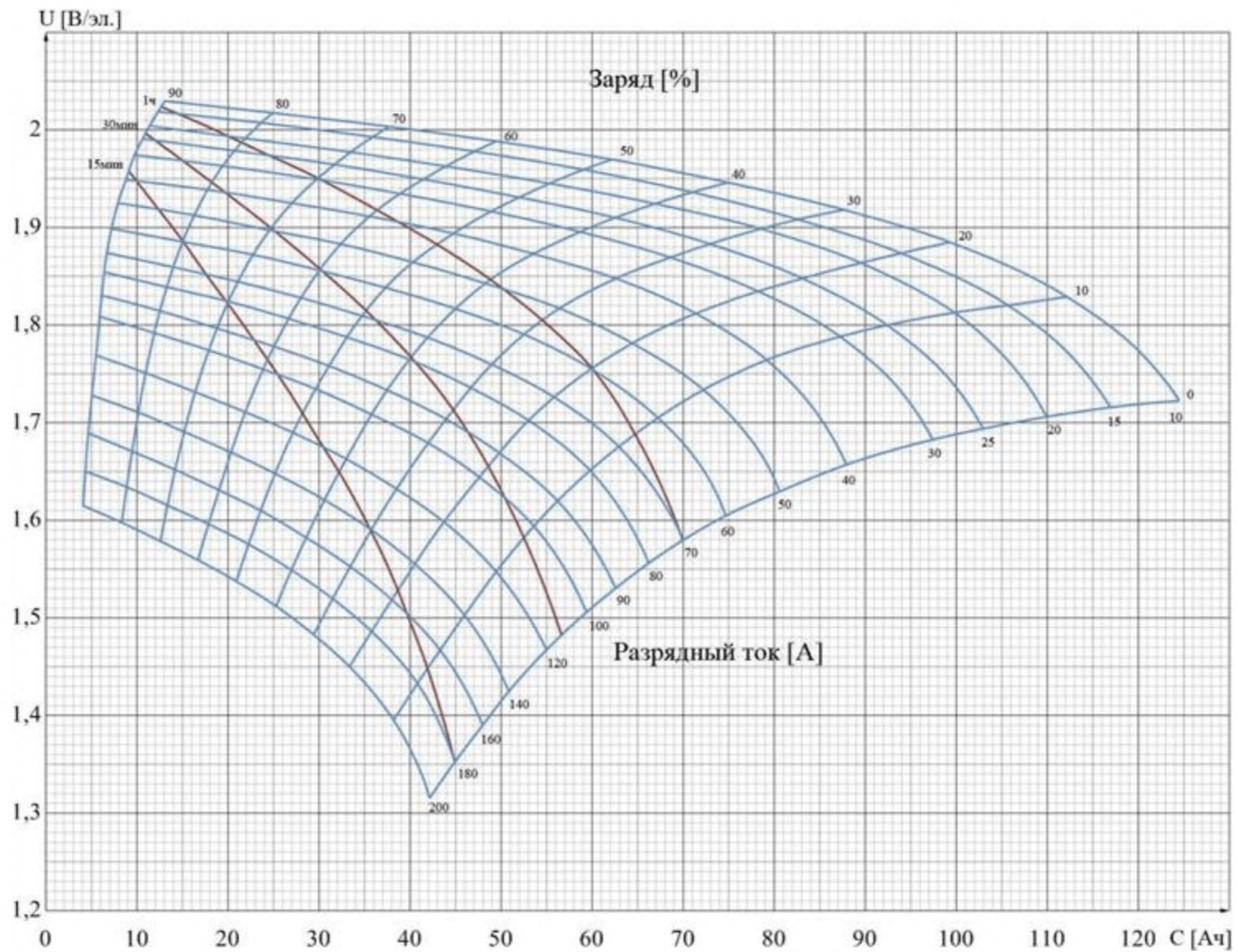
Рисунок Е.10. Разрядные характеристики АБ типа OCSM 115
