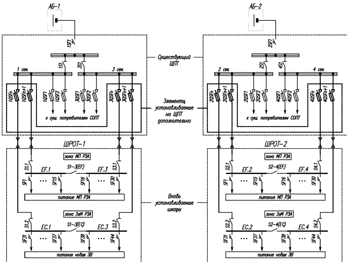
Приложение А Рисунок А7.2 Частичная реконструкция существующих СОПТ – под установку МП РЗА для количества присоединений более двух
