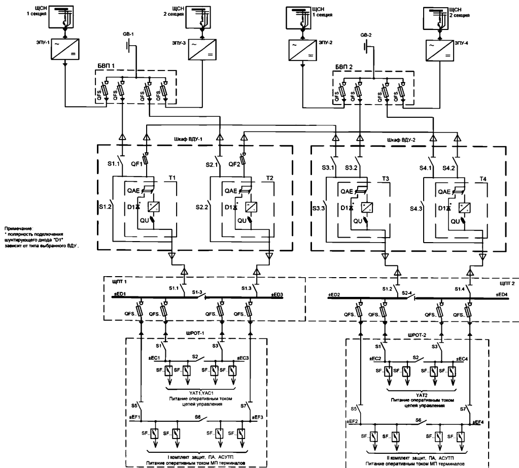
Рисунок 3. Питание устройств через ВДУ. Подключение ЗПУ через БВП. Шины ED и EF - категория питания «А1». Шины EC – категория питания «А2»
