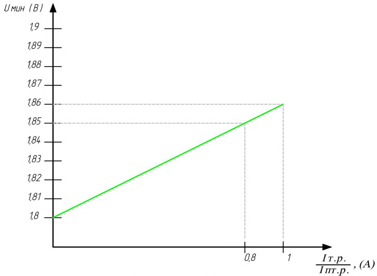
Рисунок Е.2. U_{\text{мин}} = f(I_{\text{т.р.}} / I_{\text{пг.р.}})
