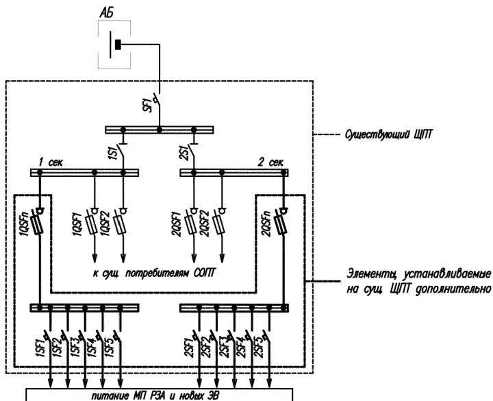
Приложение А Рисунок А7.1 Частичная реконструкция существующих СОПТ – под установку МП РЗА для одного – двух присоединений
