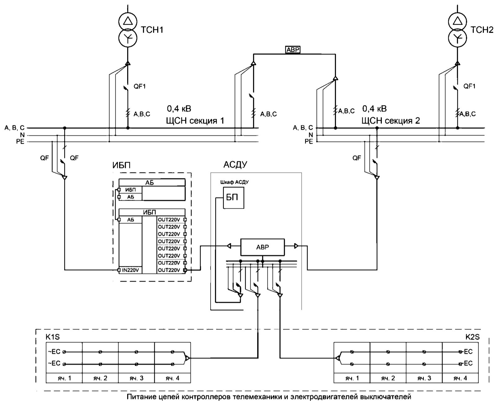
Рисунок 5. Категория питания «В2». Питание устройств переменным током с использованием ИБП
