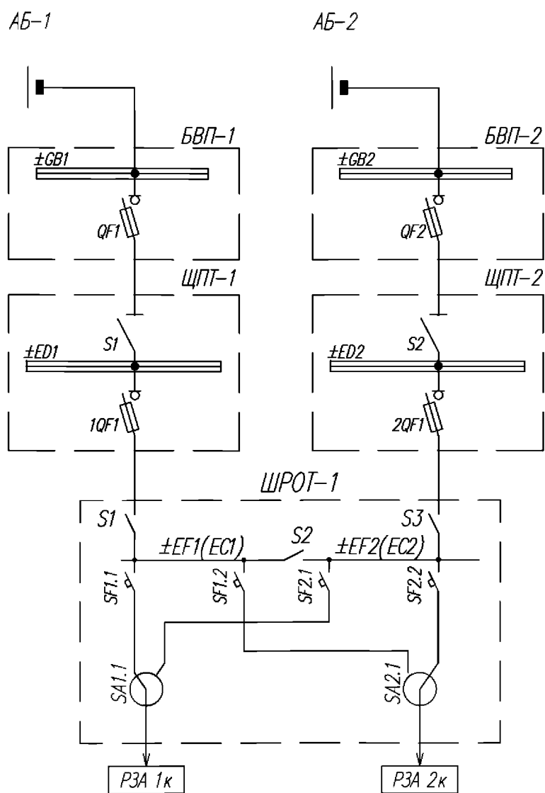
Рисунок В.1. Схема с индивидуальными ключами выбора питания для двух, резервирующих друг друга, комплектов одного присоединения.
