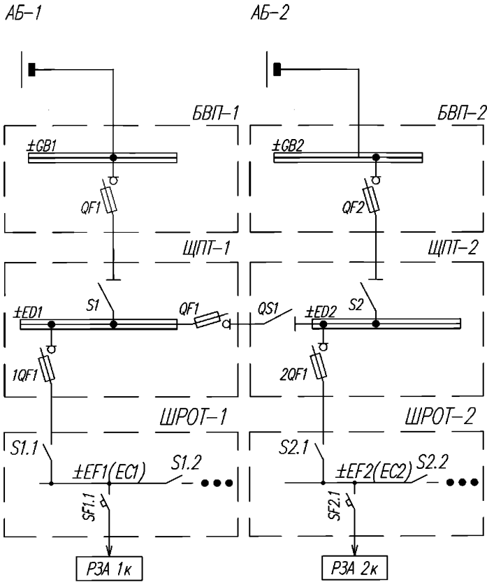
Рисунок В.3. Аппаратное резервирование, без индивидуального резервирования по питанию
