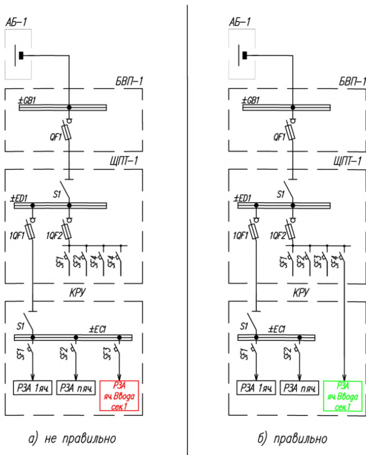
Рисунок В.6. Питание фидерных и вводных ячеек КРУ
