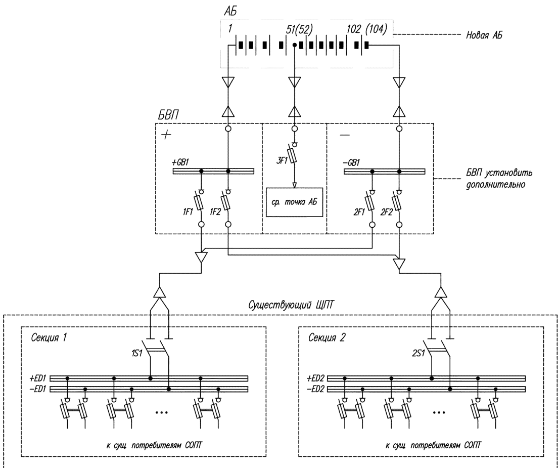
Приложение А Рисунок А7.3 Частичная реконструкция существующих СОПТ – замена АБ
