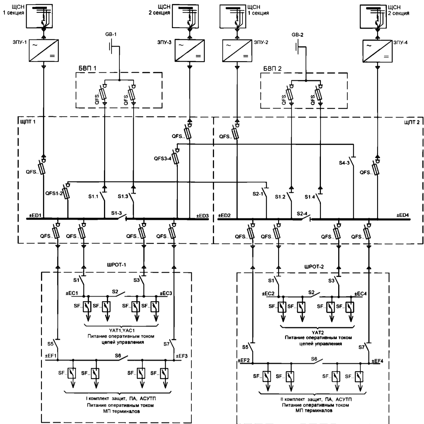
Рисунок 2. АБ подключена «напрямую» к ЩПТ. ЗПУ подключены к ЩПТ через собственные предохранители. Шины ED и EF - категория питания «А1». Шины EC - категория питания «А2»
