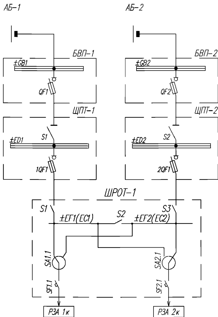
Рисунок В.2. Схема с одним защитным устройством и индивидуальными ключами выбора питания для двух, резервирующих друг друга, комплектов одного присоединения (запрещается к применению)
