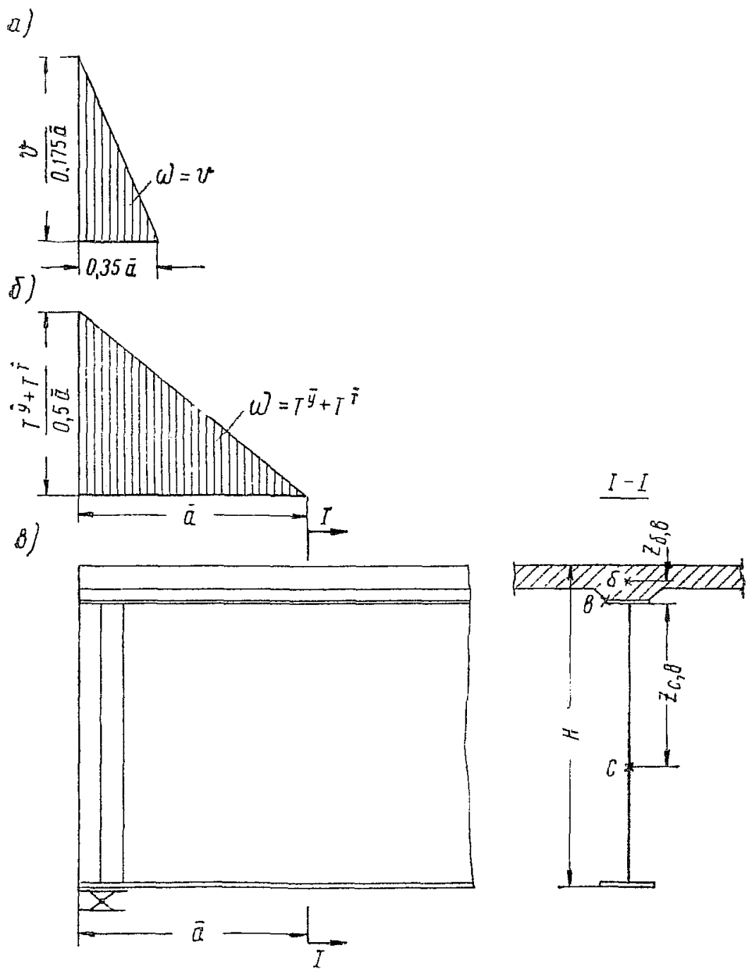
Рис. 31. Схема и эпюры к определению конечных сдвигающих и отрывающих усилий между железобетонной плитой и стальной конструкцией:
