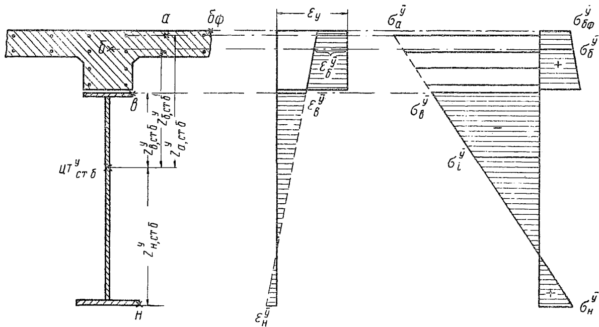
Рис. 29. Эпюры к определению внутренних напряжений от усадки бетона (ЦТ у стб — центр тяжести объединенного сечения для расчета на усадку)
