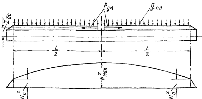
Рис. 25. Эюра усилий предварительного напряжения при обжатии железобетонной плиты горизонтальными домкратами
