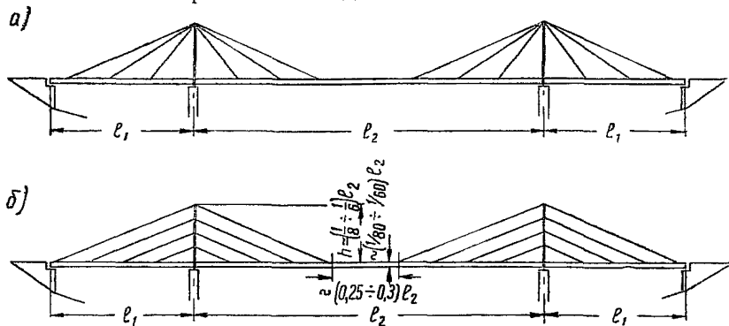
Рис. 19. Схемы вантовых мостов: а—радиально-вантовая; б—параллельно-вантовая
