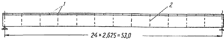
Рис. 1. Схема пролетного строения:
