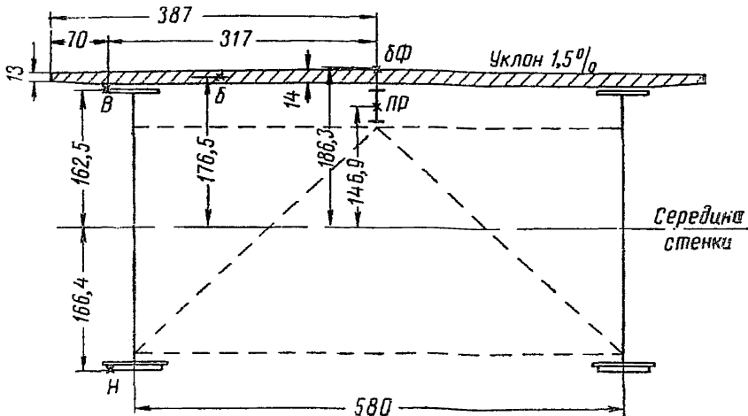
Рис. 2. Схема поперечного сечения в середине пролета
