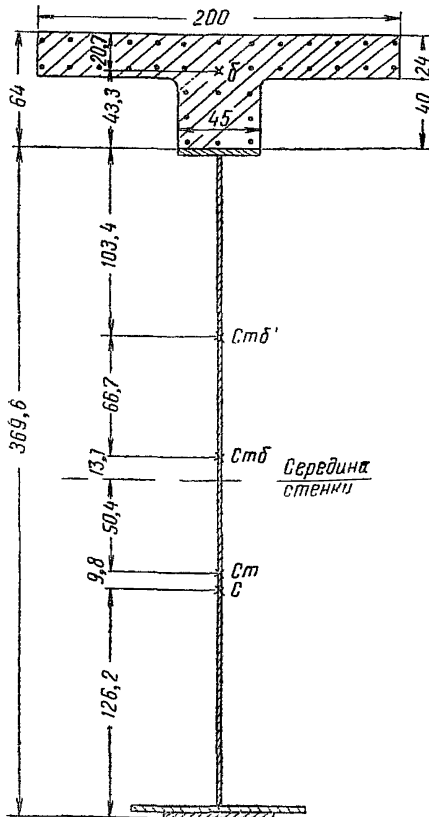
Схема поперечного сечения в середине пролета
