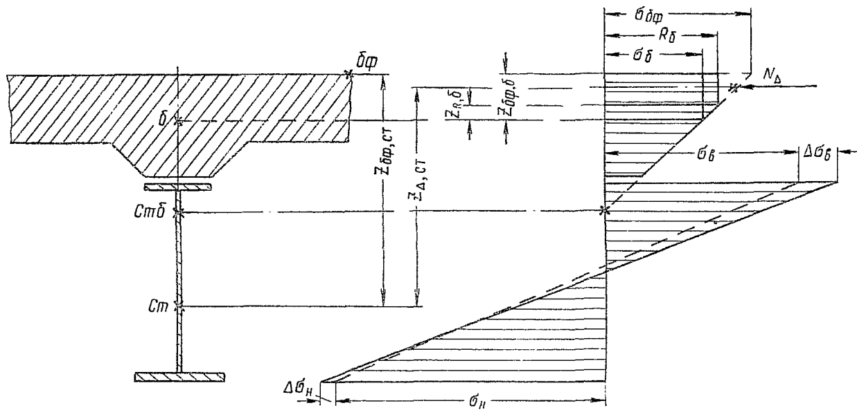
Рис. 33. Эпюры к расчету на прочность при учете развития пластических деформаций на части высоты сечения железобетонной плиты
