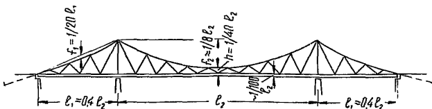
Рис. 17. Схема висячего моста с наклонными подвесками
