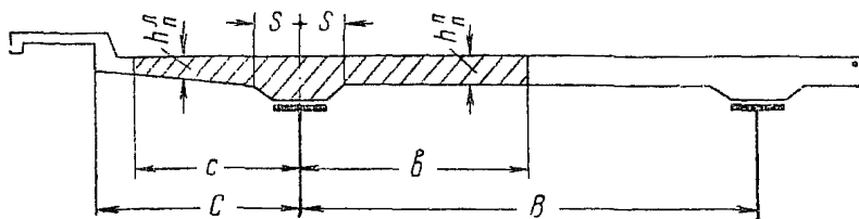
Рис. 20. Схема для определения расчетной ширины железобетонной плиты, учитываемой в составе сечения
