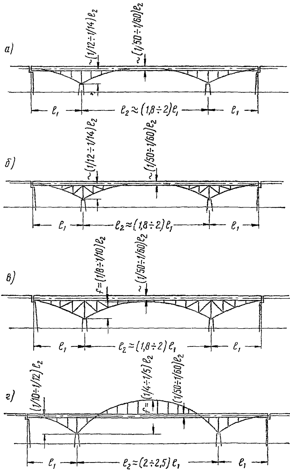
Рис. 10. Схемы подпружных пролетных строений: а—с заполнением без раскосов; б—решетчатая; в—с непрерывной подпругой; г—с ездой посередине
