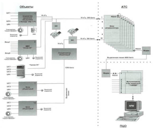
Структурная схема СПИ «Атлас-20»
