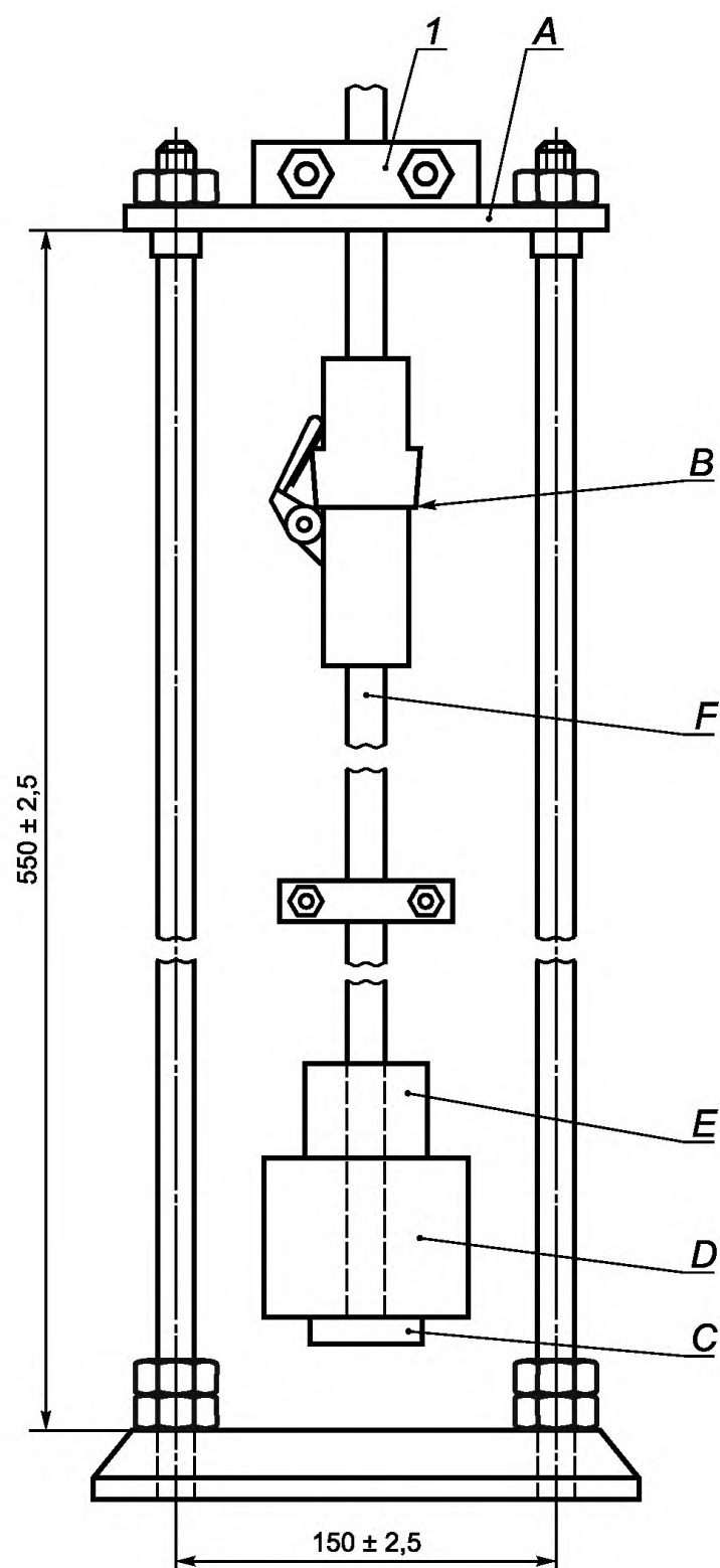
1 — кабельный зажим; A — монтажная плата; B — приборный соединитель; F — кабель; E — дополнительный груз; D — основной груз; C — держатель
