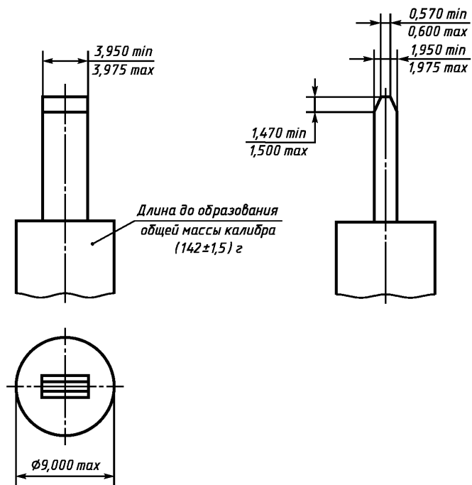
Рисунок 4 — Вытягивающий калибр (см. 13.5)
