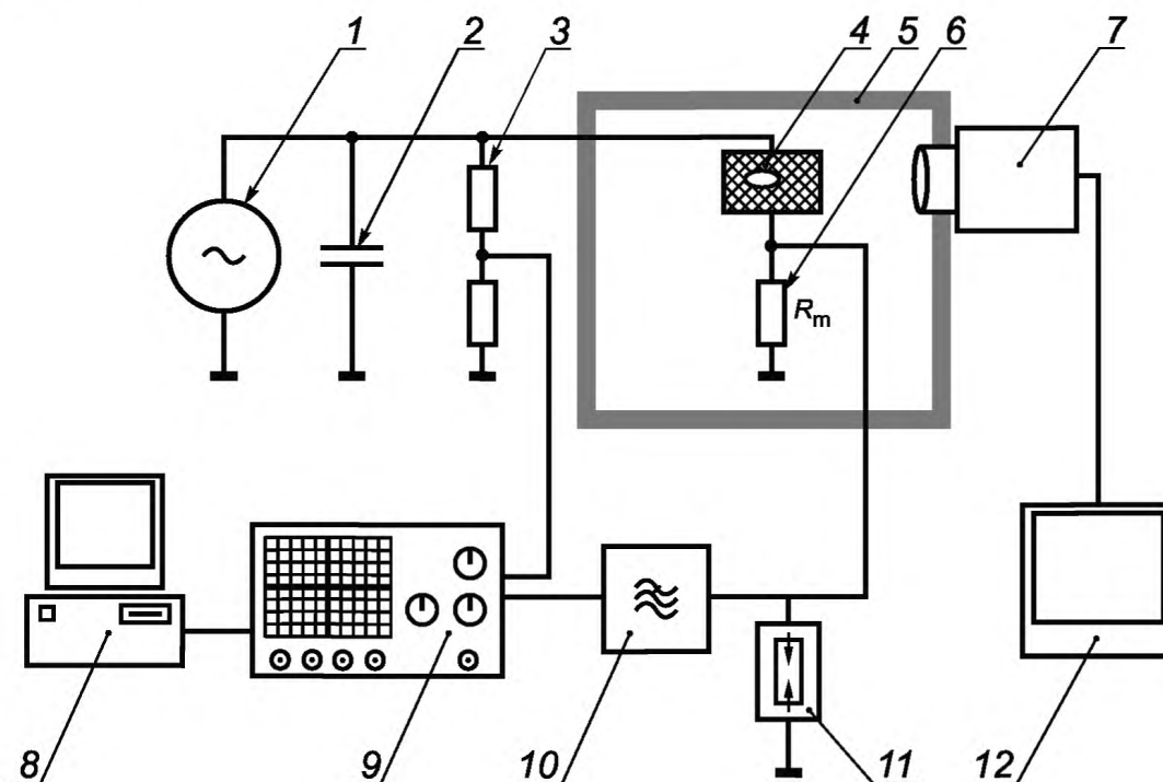
1 — источник испытательного напряжения; 2 — конденсатор связи; 3 — делитель напряжения; 4 — испытательный образец; 5 — климатическая камера; 6 — измерительный импеданс R_m ; 7 — видеокамера; 8 — компьютер; 9 — цифровой запоминающий осциллограф; 10 — полосовой фильтр; 11 — защита от перенапряжений; 12 — монитор
