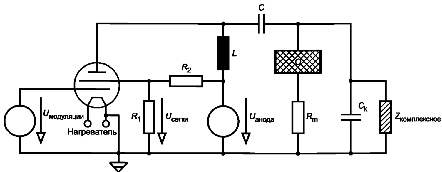
Рисунок D.2 — Высокочастотный генератор большой мощности [5] и [6]
