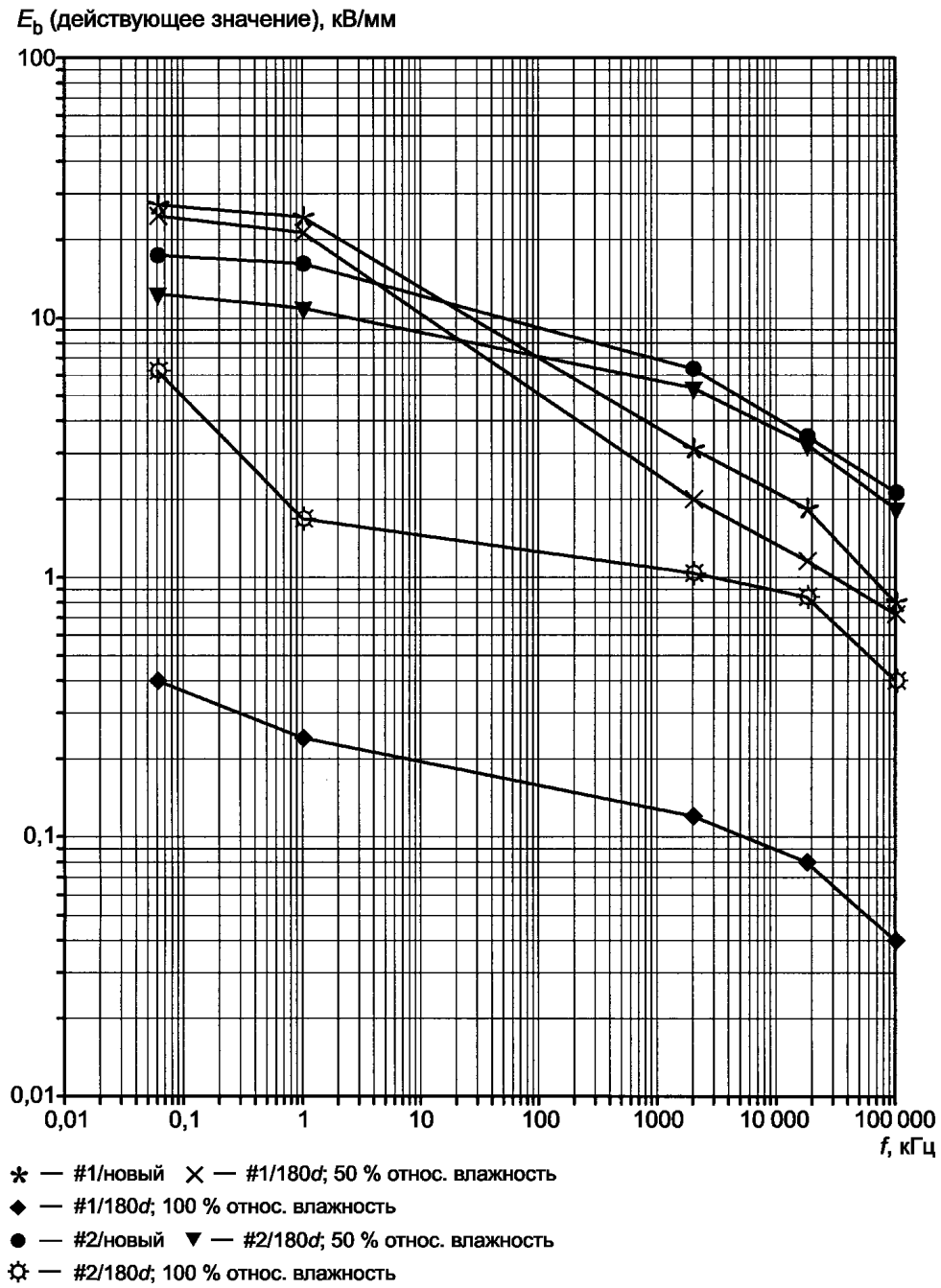
Рисунок С.4 — Высокочастотный пробой твердой изоляции, влияние влажности; условия при 50 °С: #1: наполненный слюдой фенол, d = 0,75 мм; #2: ламинат из кремниевого стекла, d = 0,75 мм [19]
