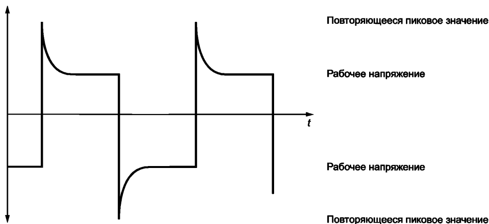
Рисунок 4 — Периодическое импульсное напряжения (см. IEC 60664-1)
