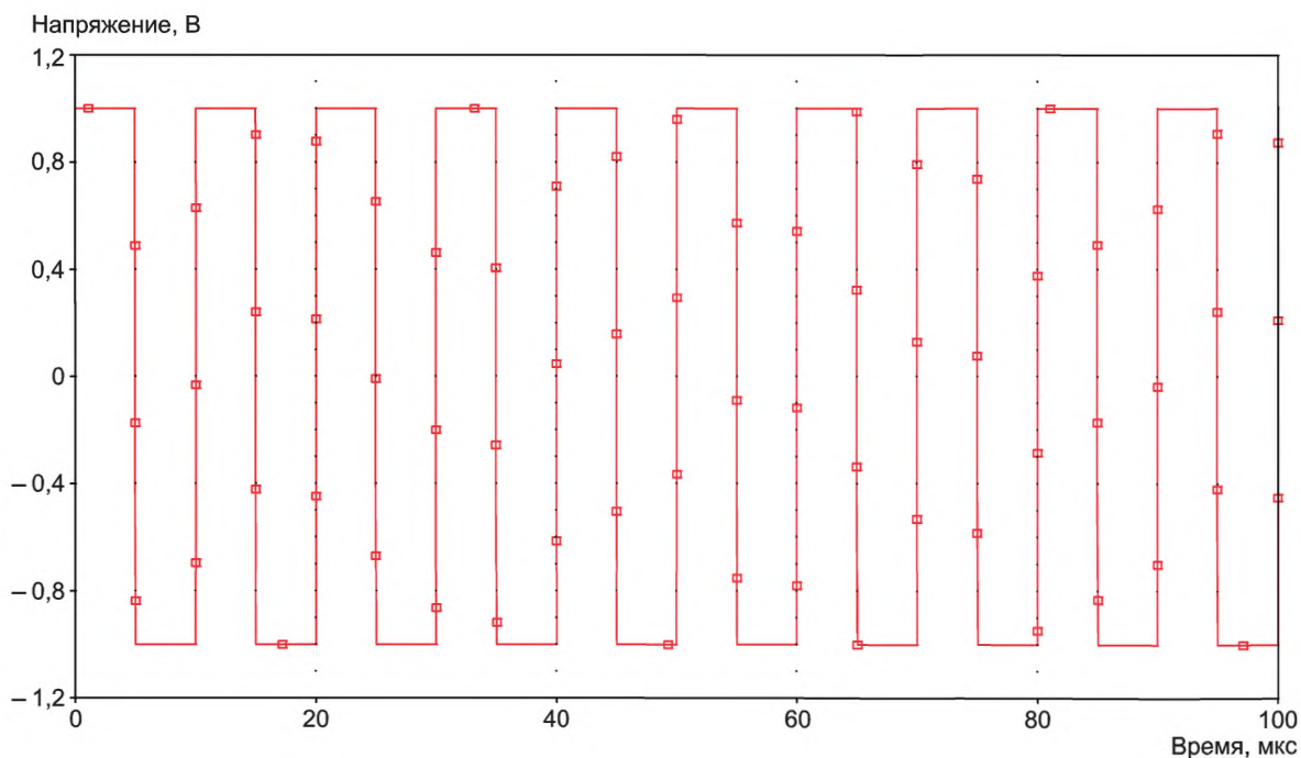
Рисунок E.1 — Периодические импульсы напряжения, прямоугольная форма волны
