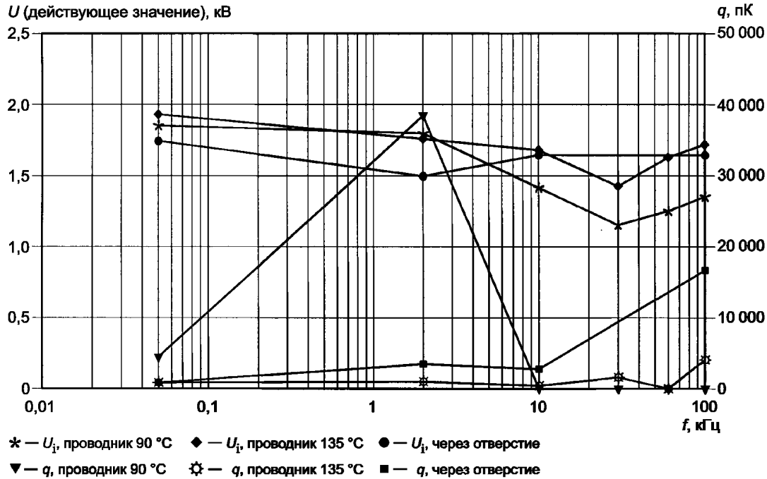
Рисунок D.11 — Испытание ЧП покрытых печатных плат; U_i , d = 0,2 мм [30]
