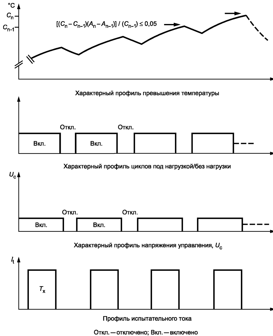
Рисунок F.1 — Профиль испытания на тепловую стабильность
