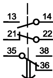
Три контактных элемента
