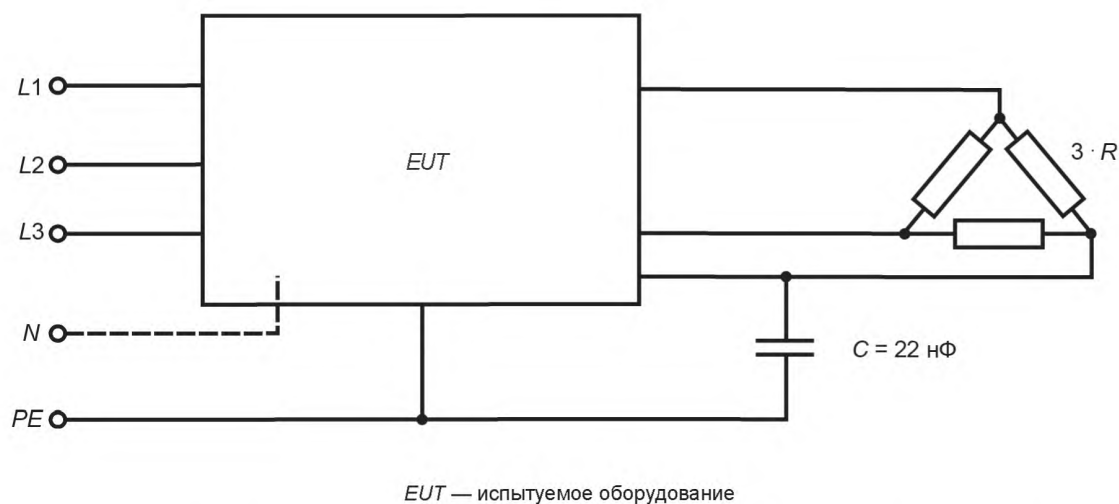
Рисунок I.2 — Испытательная цепь для измерения эталонного (опорного) потенциала, вызванного нагрузкой, — трехфазный выход
