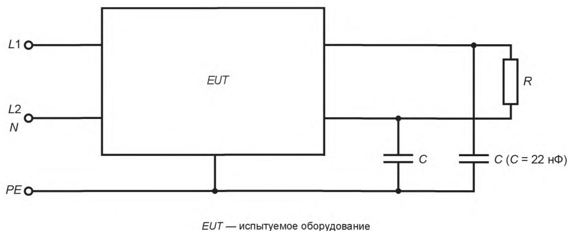
Рисунок I.1 — Испытательная цепь для измерения изменения эталонного (опорного) потенциала, вызванного нагрузкой, — однофазный выход
