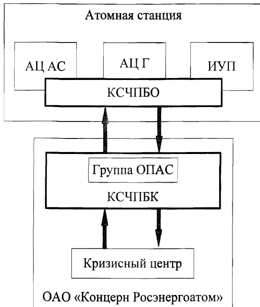
Рисунок 5.1 - Схема взаимодействия АЭС с КЦ Концерна при ЧС
