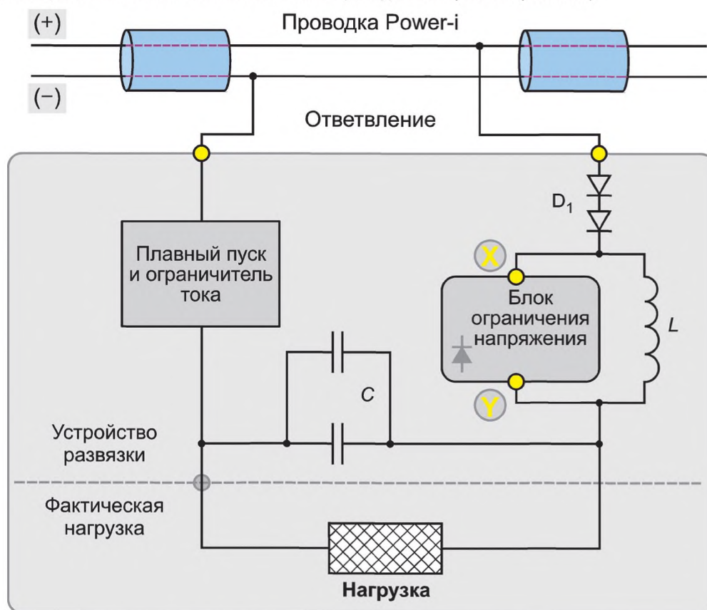
Рисунок С.2 — Пример обычного полевого устройства Power-i
