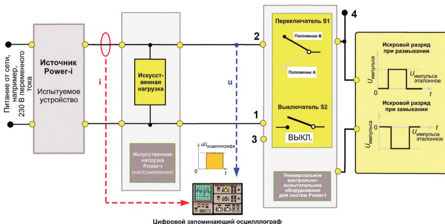
Рисунок А.4 — Принцип действия оборудования при определении времени отклика t_{\text{отклика источника}}
