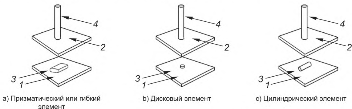
Рисунок 4 — Примеры установки для испытания на раздавливание
