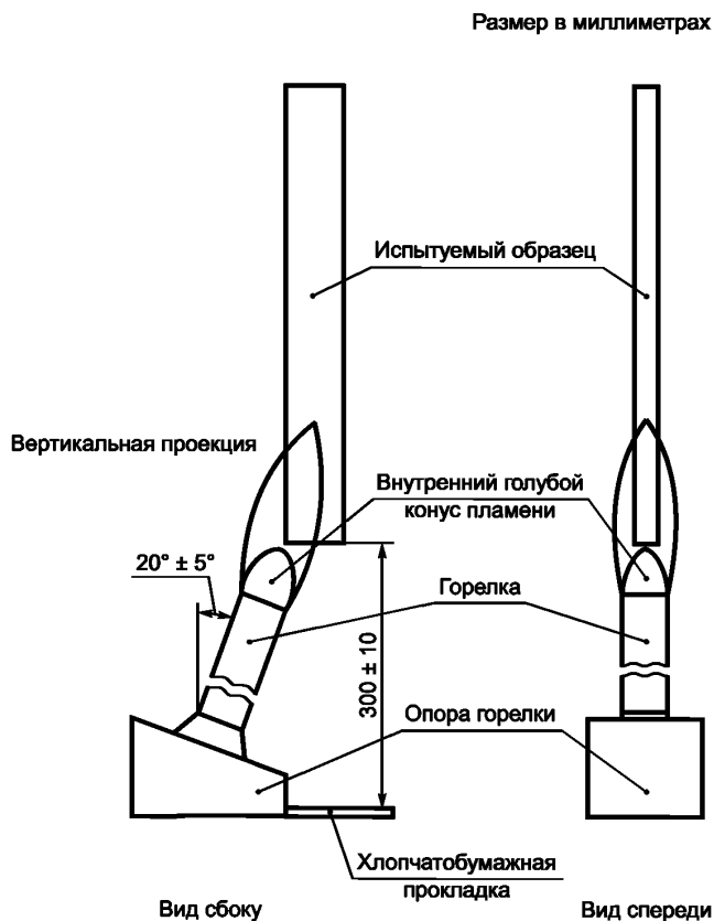
Рисунок 1 — Испытание вертикального горения для брускового испытуемого образца
