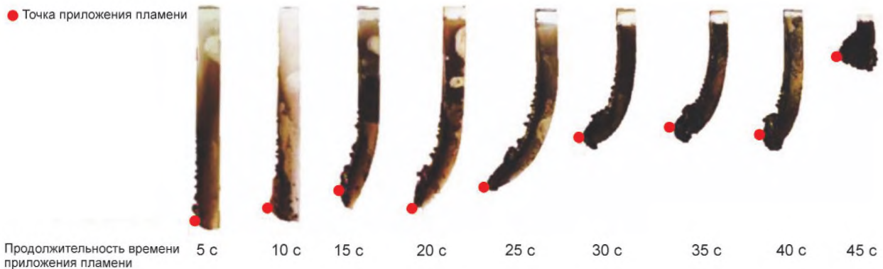
Рисунок А.1 — Точки приложения пламени для образца, который деформируется динамически
