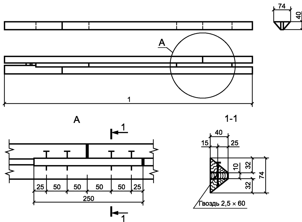
Рисунок А.1 — Пример стыкования брусков обвязки
