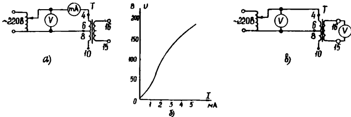
Рис. 27. Схемы проверки трансформатора реле РИС-Э2М, РИС-Э2М-0,2:
