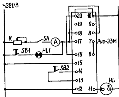
Рис. 24. Схема настройки реле РИС-ЭЗМ
