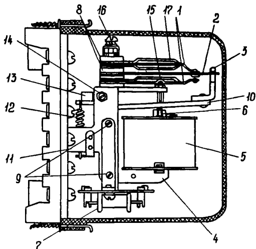
Рис. 5. Общий вид реле РП-220:
