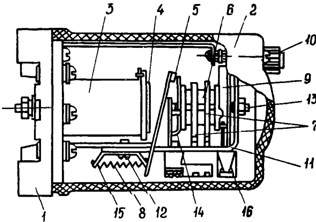
Рис. 12. Общий вид реле РУ-21:
