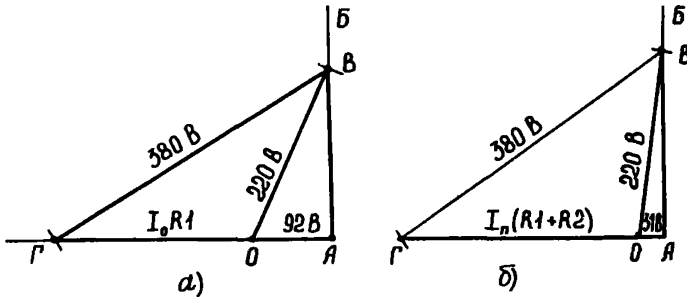
Рис. П1.4. Графическое определение сопротивления:
