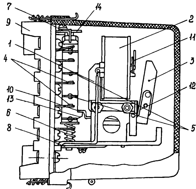
Рис. 3. Общий вид реле РП-25:
