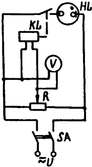
Рис. 16. Схема проверки напряжения срабатывания и возврата реле
