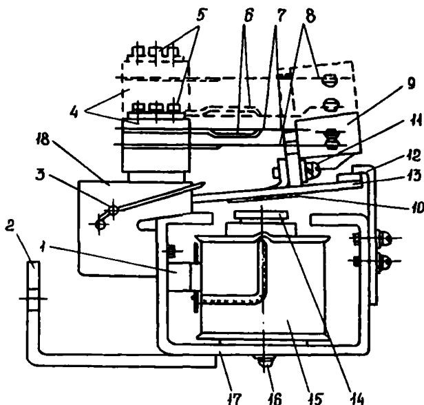
Рис. 6. Общий вид реле РПУ-1-010:
