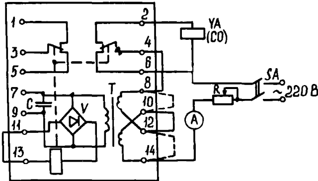
Рис. 21. Схема проверки надежности работы контактной системы реле РП-341
