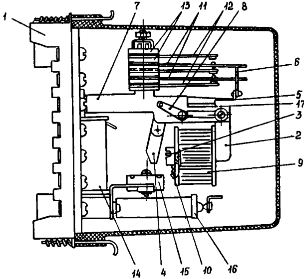
Рис. 9. Общий вид реле РП-321:
