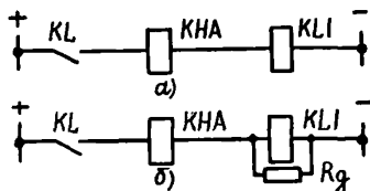
Рис. П1.1. Расчетные схемы для выбора указательного реле:
