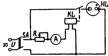
Рис. 17. Схема проверки тока срабатывания и возврата реле
