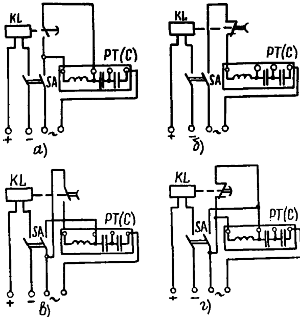
Рис.19. Схемы измерения:
