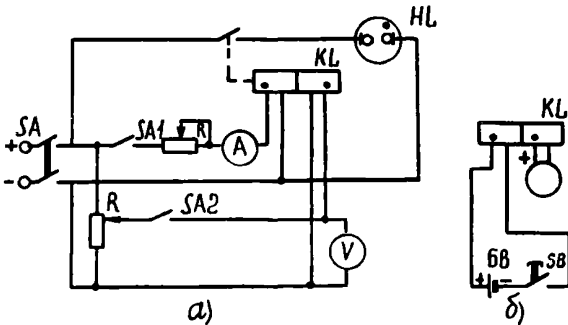
Рис. 18. Схемы проверки однополярных выводов реле:
