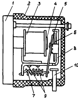
Рис. 13. Общий вид реле ЭС-41:
