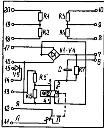
Рис. 15. Принципиальная схема реле РИС-Э3М
