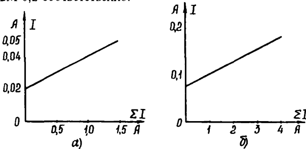
Рис. 22. Зависимость значений импульса тока срабатывания:
