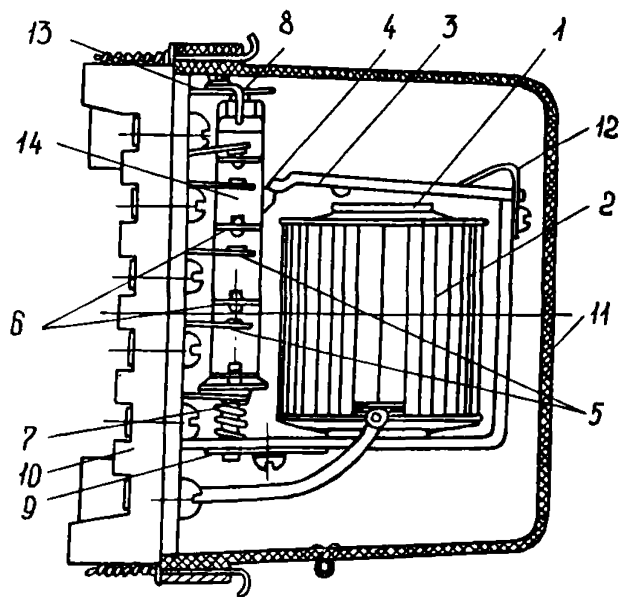
Рис. 2. Общий вид реле РП-23, РП-232, РП-233:
