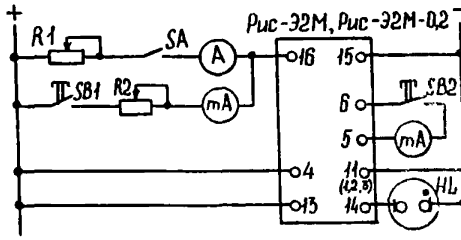
Рис. 23. Схема настройки реле РИС-Э2М, РИС-Э2М-0,2
