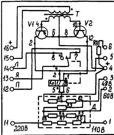
Рис. 14. Принципиальная схема реле РИС-Э2М
