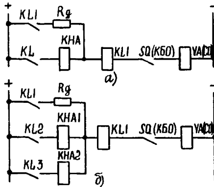
Рис. П1.2. Схема выходных цепей защиты:
