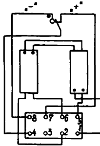
Рис. 26. Схема внутренних соединений поляризованного реле ТРМ-Т
