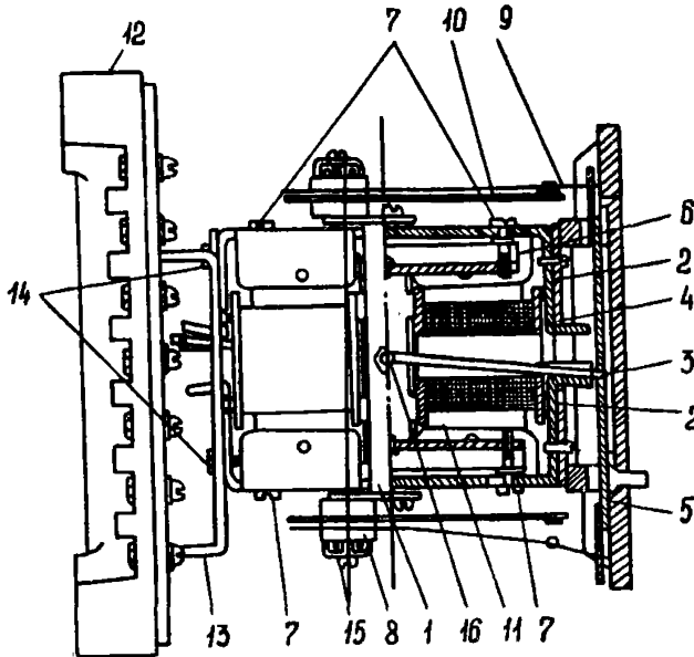
Рис. 10. Общий вид реле РП-11, РП-12:
