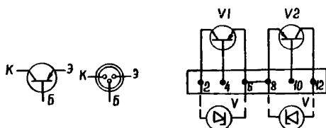
Рис. 28. Цоколевка и монтажная планка крепления транзисторов V1, V2 реле РИС-ЭЗМ, РИС-ЭЗМ-0,2
