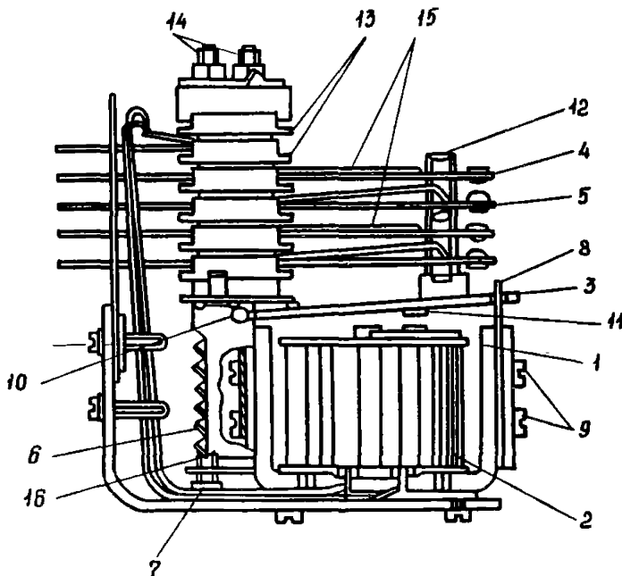
Рис. 7. Общий вид реле МКУ-48:
