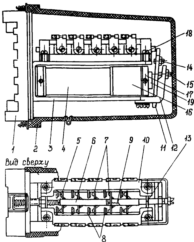
Рис. 4. Общий вид реле РП-251:
