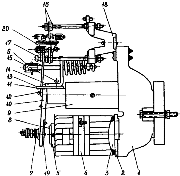
Рис. 11. Общий вид реле РЭВ-883, РЭВ-884:
