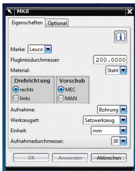
Рисунок 17 — Экранное окно ввода проектировщика
