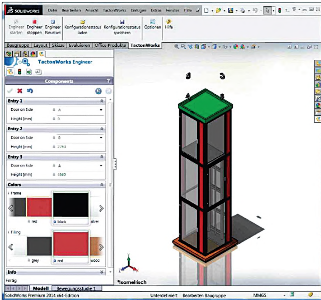
Рисунок 21 — Готовая сконфигурированная подъемная система
