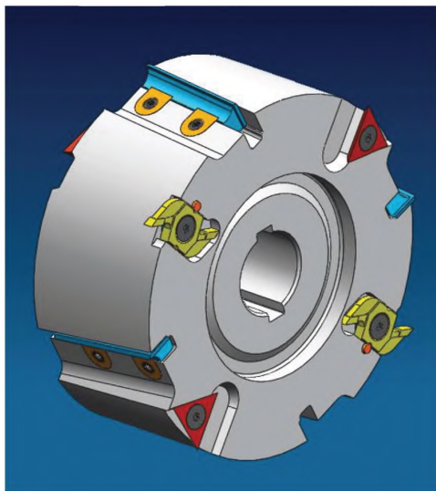
Рисунок 16 — Конфигурируемая режущая головка
