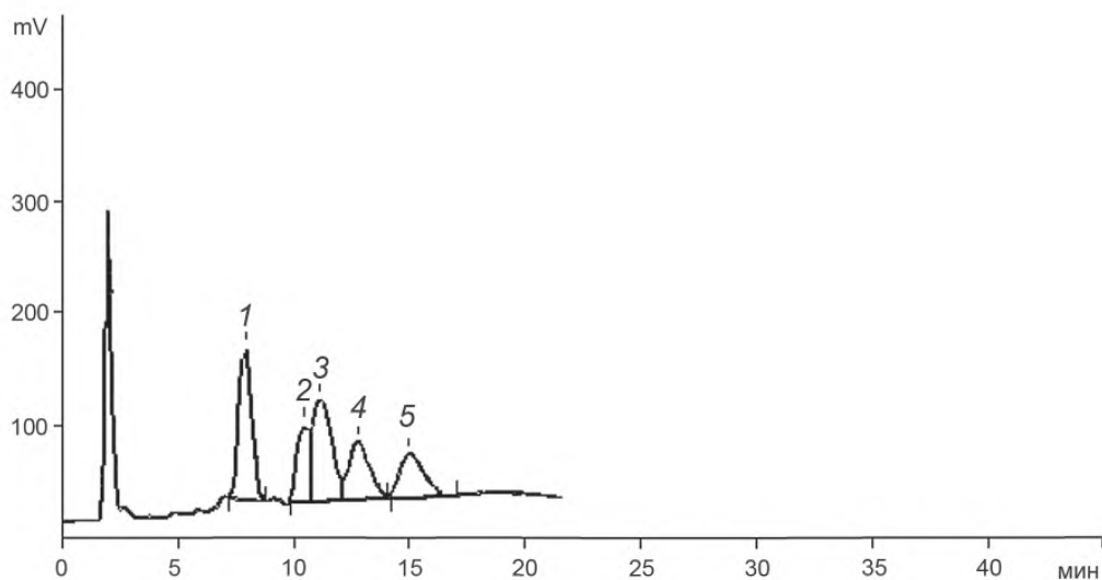
Рисунок 1 — Хроматограмма смеси стандартов стерина
