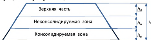
Рисунок 2 – Поперечный профиль насыпи из грунта повышенной влажности с выделением неконсолидируемой (пассивной) и консолидируемой (активной) зон
