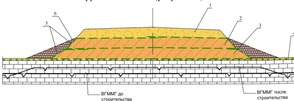
Рисунок 10 – Насыпь из переувлажненных глинистых грунтов на основаниях III-IV категорий просадочности
