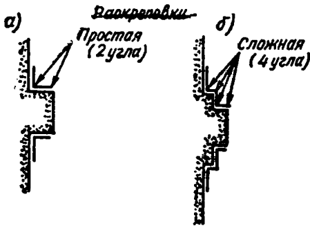
Рис. 2. Раскреповки
