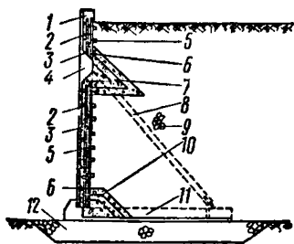
Рис. 6. Вертикальный обратный фильтр
