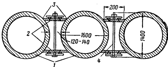
Рис. 17. Устройство подводной опалубки для омоноличивания зазоров между оболочками (план)
