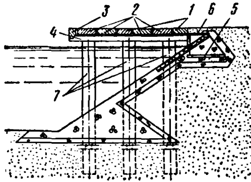
Рис. 8. Поперечный разрез причала на колоннах-оболочках диаметром 1,6 м
