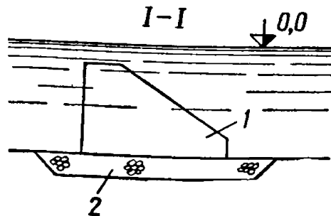
Рис. 21. Подводный волнолом из массивовой кладки
