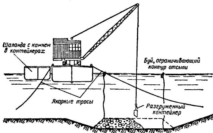
Рис. 23. Отсыпка камня из контейнеров в постель сооружения
