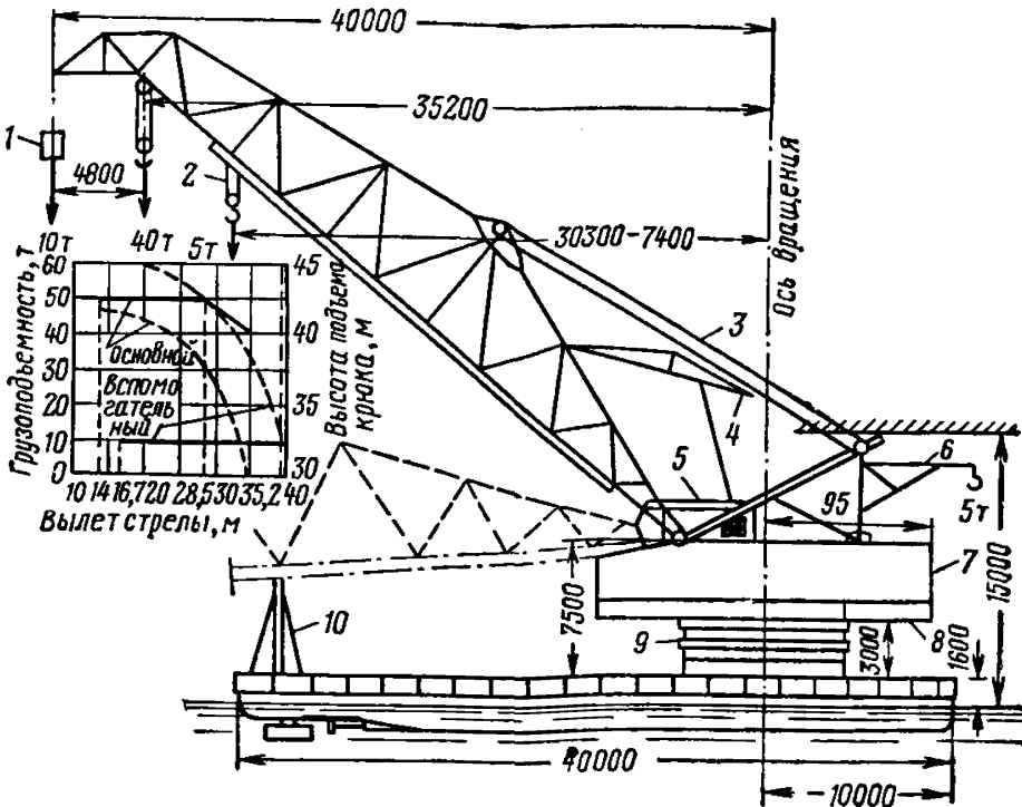
Рис. 28. Схема плавучего 50 т крана «Блейхерт»
