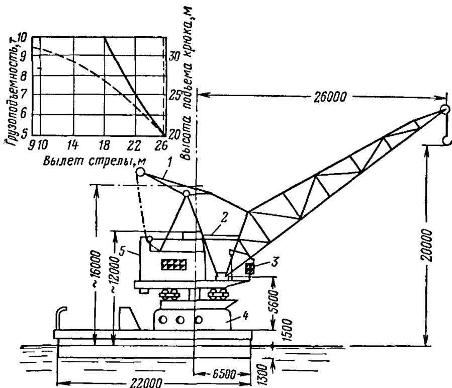
Рис. 26. Схема универсального плавучего крана «Валмет»
