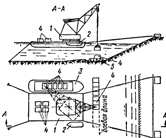
Рис. 3. Схема монтажа стенки из правильной массивной кладки
