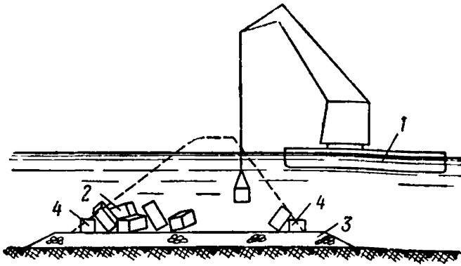
Рис. 19. Оградительное сооружение из наброски бетонных массивов
