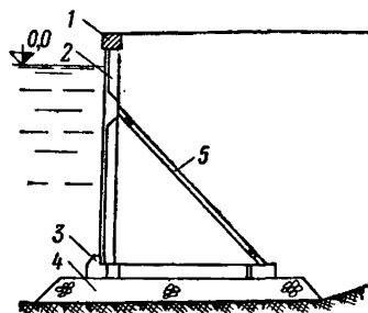
Рис. 2. Поперечный разрез набережной уголкового профиля
