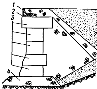
Рис. 1. Поперечный разрез набережной из правильной массивовой кладки
