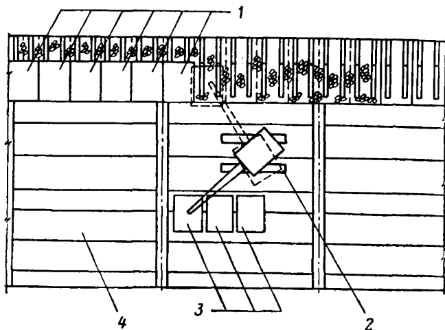
Рис. 15. Схема установки плит, перекрывающих короба тылового сопряжения
