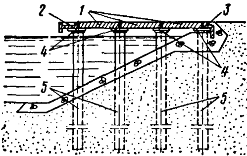
Рис. 9. Поперечный разрез причала на колоннах-оболочках диаметром 1,2 м
