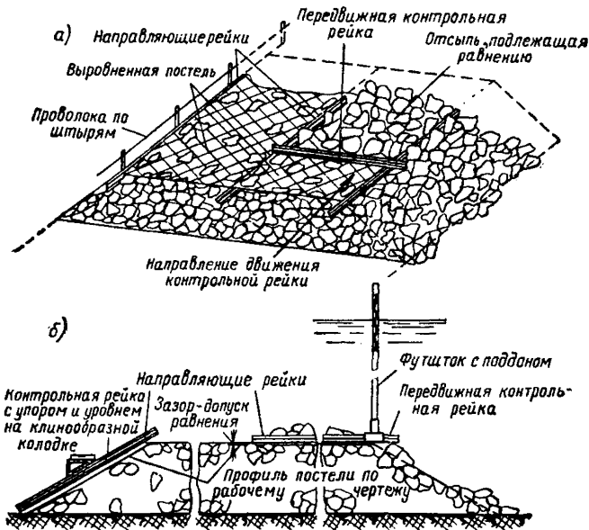
Рис. 24. Весьма тщательное и тщательное равнение постели
