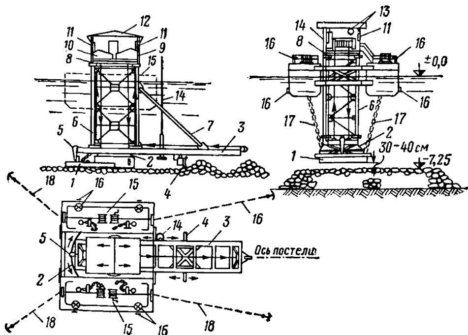
Рис. 25. Механический подводный планировщик
