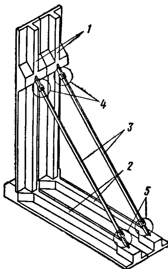
Рис. 4. Плиты углового блока
