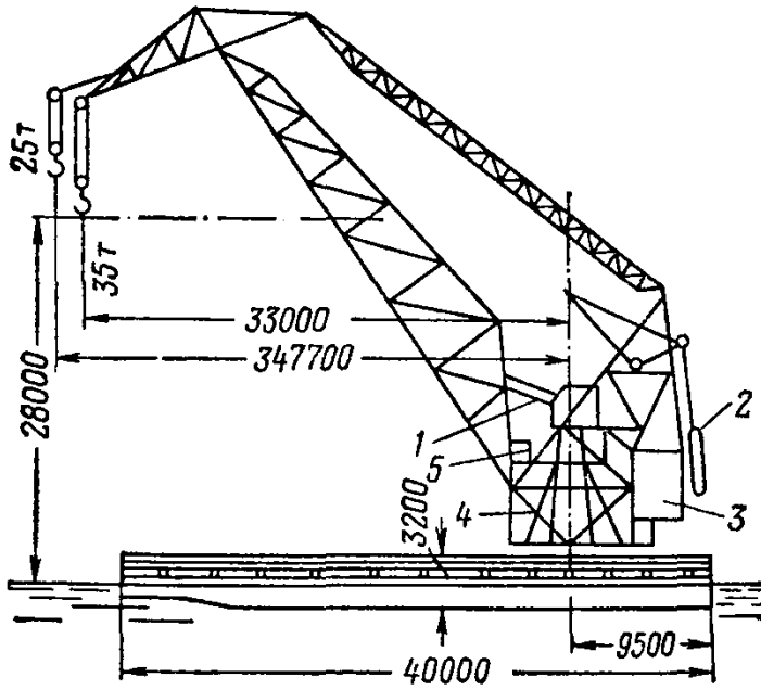
Рис. 29. Схема плавучего 100-т крана «Ганц».
