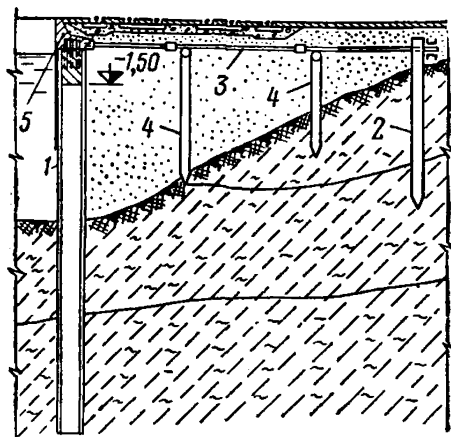
Рис. 16. Поперечный разрез причала
