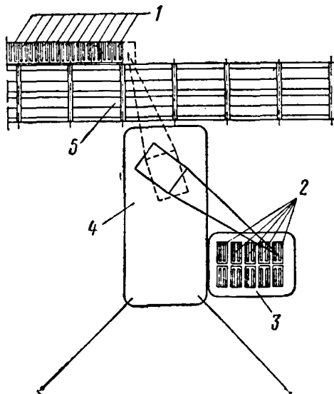
Рис. 14. Схема установки коробов тылового сопряжения
