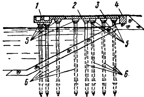
Рис. 10. Поперечный разрез причала на призматических сваях
