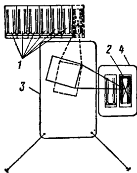
Рис. 7. Схема монтажа причальной набережной из угловых блоков с внутренним анкером
