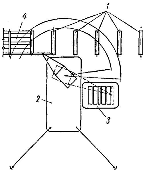
Рис. 13. Схема установки бортовых балок и пролетных плит верхнего строения
