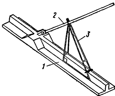
Рис. 5. Плита с прикрепленной анкерной тягой
