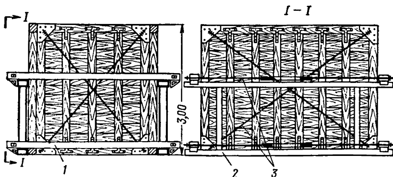
Рис. 22. Деревянно-металлическая опалубка обыкновенных массивов 1 — металлическая балка; 2 — металлическая плоская рама; 3 — стяжки
