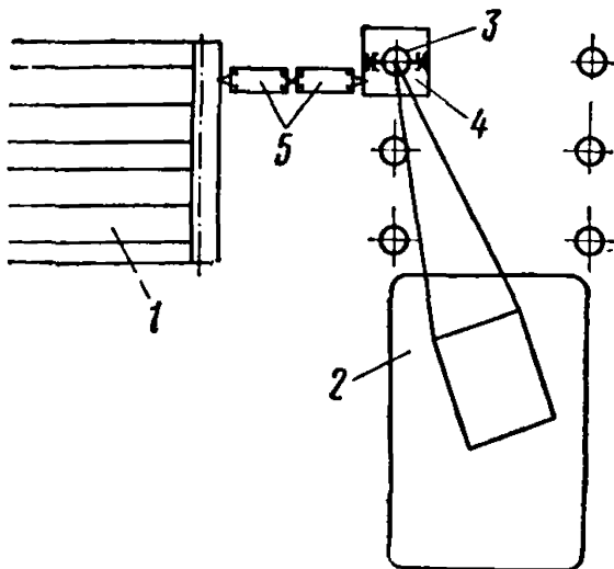
Рис. 11. Установка железобетонных дниц в полости колонн-оболочек
