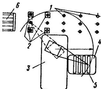
Рис. 12. Схема установки ригелей на свайные ряды из колонн-оболочек
