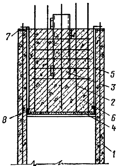
Рис. 18. Бетонирование верха внутренней полости колонн-оболочек
