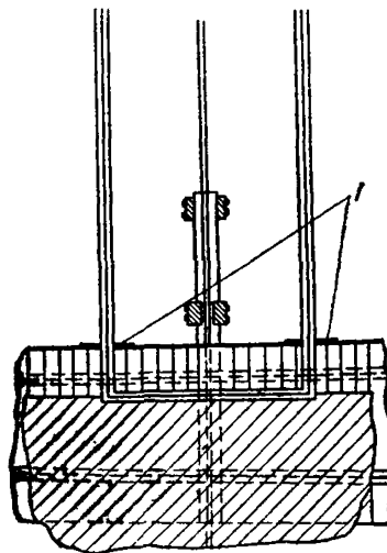
Рис. 37. Установка временной коробки, попадающей на домкратную раму 1 — доски, снимаемые при установке первой распорки
