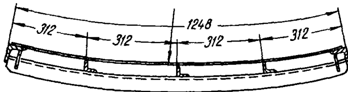
Рис. 28. Щит наружный стальной 1 — обвязка вертикальная; 2 — обвязка горизонтальная; 3 — кружало; 4 — ребро жесткости; 5 — листовая сталь
