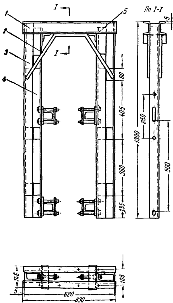
Рис. 32. Рама гидродомкрата
