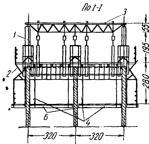
Рис. 33. Схема стальной опалубки рабочей башни с опорными фермами
