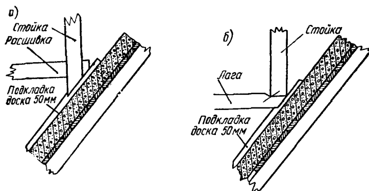
Рис. 18. Установка дополнительной стойки на стенные бункера а — на стенку бункера; б — на лагу
