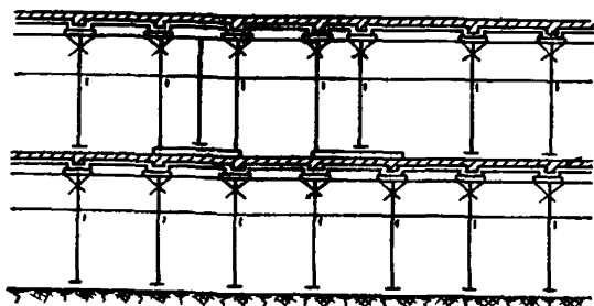
Рис. 3. Схема лесов под опалубку перекрытий, расположенных на высоте до 6 м
