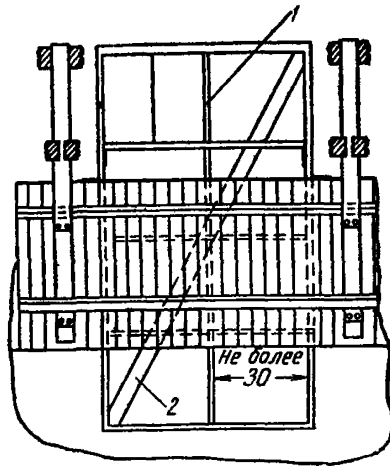
Рис. 36. Установка временной коробки при расположении между домкратными рамами 1 — вертикальные распоры; 2 — распорки из досок
