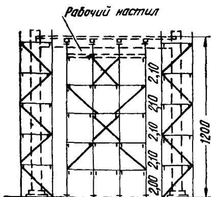
Рис. 4. Схема лесов под опалубку перекрытий, расположенных на высоте более 6 м
