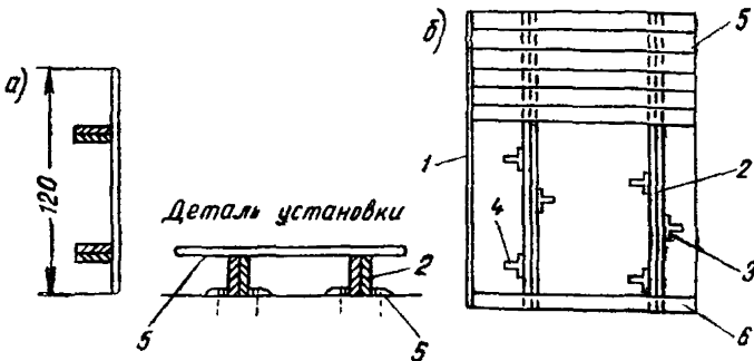
Рис. 27. Сборка деревянного наружного прямолинейного щита а — щит; б — установка для изготовления щитов; 1 — контрольная рейка; 2 — ребра; 3 — клинья; 4 — бобышки; 5 — клепка; 6 — контрольная клепка
