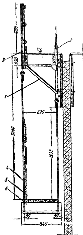
Рис. 30. Подвесные подмости на металлических подвесках и козырек с ограждением
