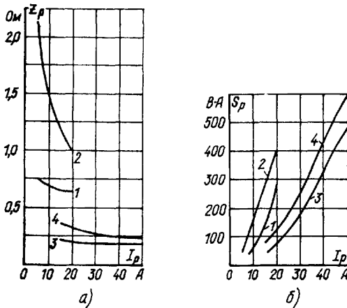
Рис.Ш.4. Характеристики реле РТМ Рижского опытного завода "Энергоавтоматика":
