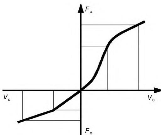
Рисунок 4 — Зависимость сопротивления амортизатора от скорости перемещения поршня
