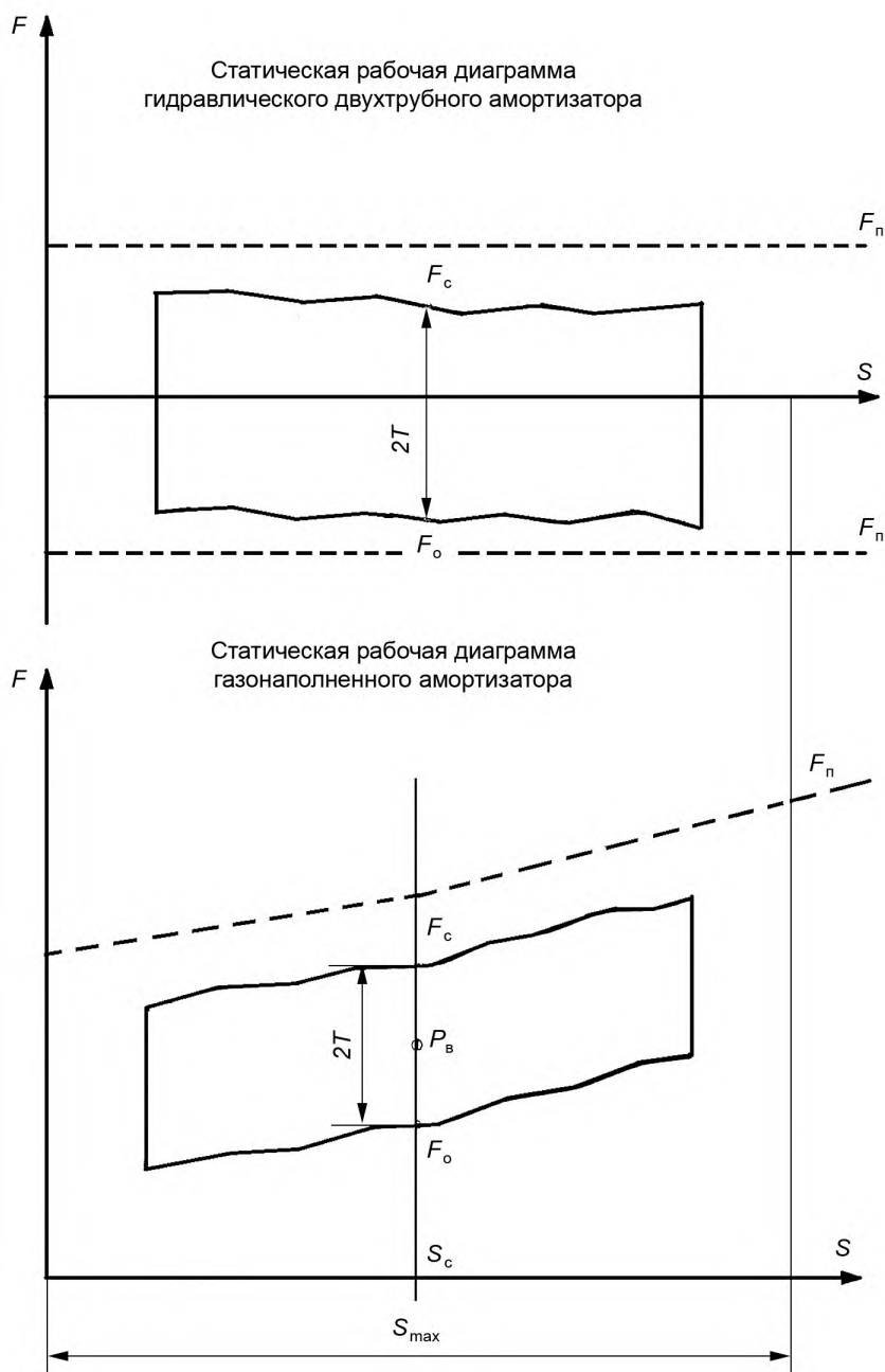
Рисунок 1 — Статические рабочие диаграммы амортизаторов
