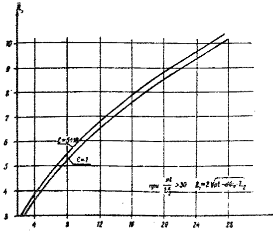
Рис.37. График для определения величины R_1 .
