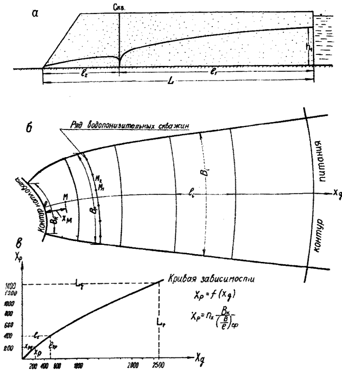
Рис.63. Схема к расчету ряда водопонижительных скважин вблизи карьера.
