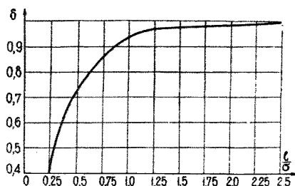
Рис.46. График для определения расхода горизонтальных скважин.
