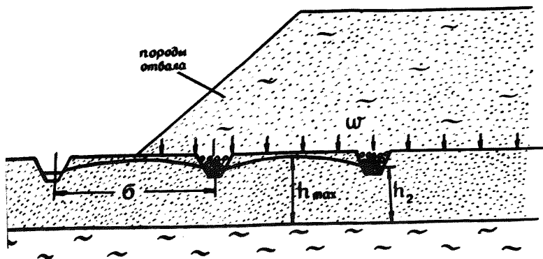
Рис.40. Схема к расчету систематического дренажа отвалов.
