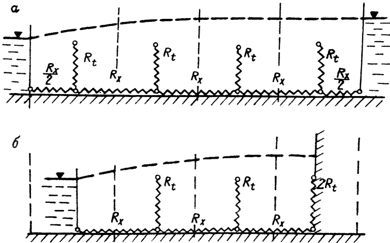
Рис.53. Схема к разбивке поля фильтрации при моделировании неустановившегося режима.
