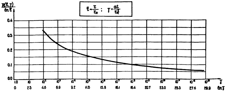
Рис.16. График функции R(\bar{r}, r) .
