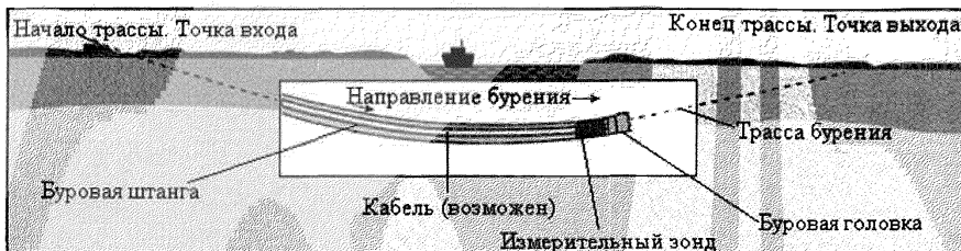
Рисунок 8.3 – Направленное бурение пилотной скважины
