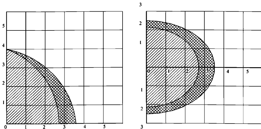
Рис.М.2. Диаграмма распыла НС-145 под углом 90^{\circ} к горизонту
