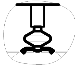
Вариант 2. Установка распылителей за фальшпотолком (работа сквозь перфорацию потолка)
