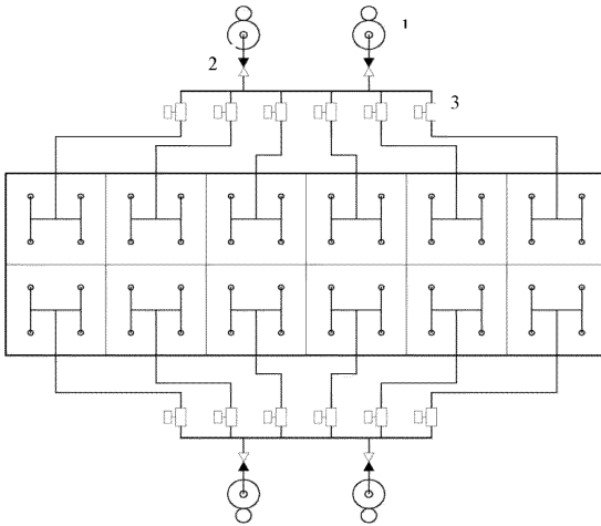
Рис.6.9 Схема позонной защиты помещений неограниченной площади модулями «Гарант-160»
