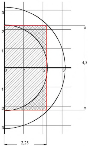
Рис. 6.3. Зона тушения НС-360(при расположении на вертикальной поверхности-стене).
