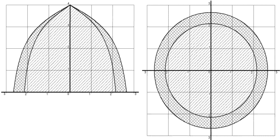
Рис. И.5 Конфигурация распыла одиночного распылителя НС-360 при расположении распылителя к защищаемой горизонтальной поверхности вертикально(симметричный распыл).
