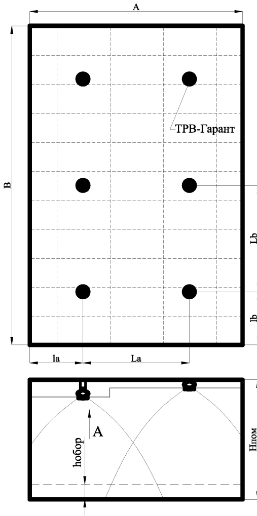
Вариант 1. Установка распылителей ниже уровня фальшпотолка
