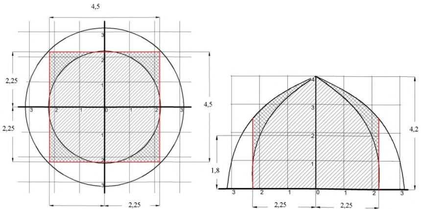
Рис.6.2. Диаграмма распыла и площади(зоны) тушения насадка НС-360.
