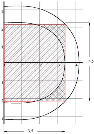
Рис.6.5. Зона тушения НС-390-С(при расположении на вертикальной поверхности-стене).
