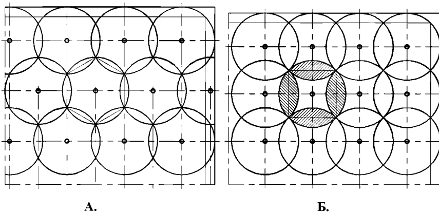
Рис.В.1. Способы взаимной расстановки модулей: А-шахматный; Б-квадратный.
