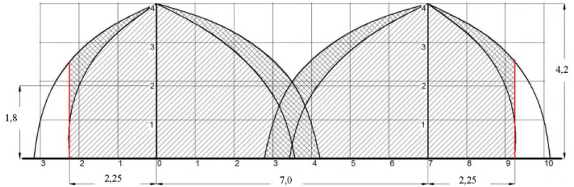
Рис.6.5. Зона тушения НС-390-С(при расположении на вертикальной поверхности-стене).
