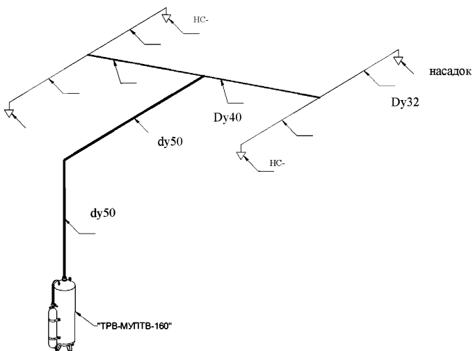
Рис.6.1 Схема технологической части установки «ТРВ Гарант-160».
