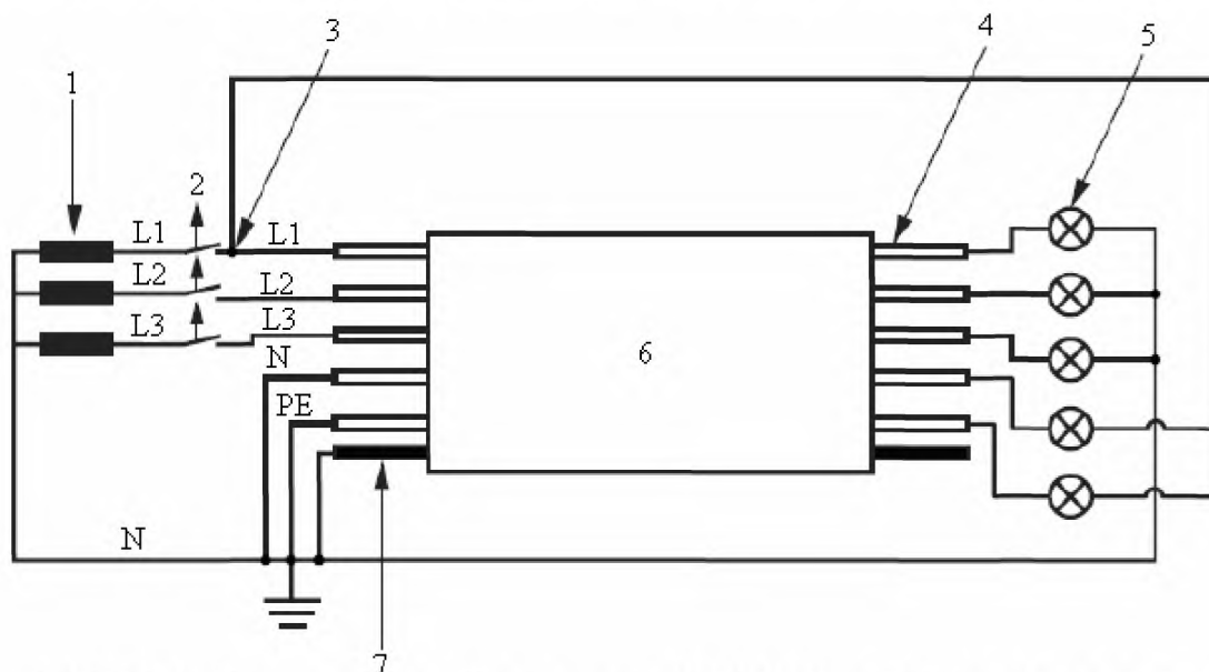
L1, L2, L3 - фазовые провода (если имеются L2, L3); N - нейтральный провод (если имеется); PE - защитное заземление (если имеется); 1 - трансформатор; 2 - плавкий предохранитель, (2 А); 3 - соединение к фазе L1 (или L2 или L3); 4 - испытательный провод или группа; 5 - нагрузка и индикаторное устройство; 6 - образец для испытания; 7 - металлический экран (если имеется).
