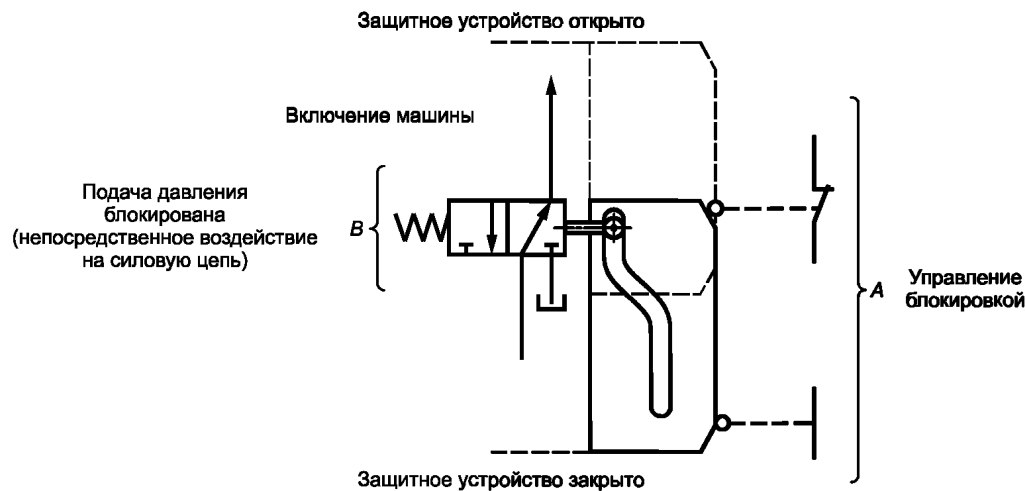
Рисунок L.3 — Комбинированное (электрическое и гидравлическое) блокировочное устройство
