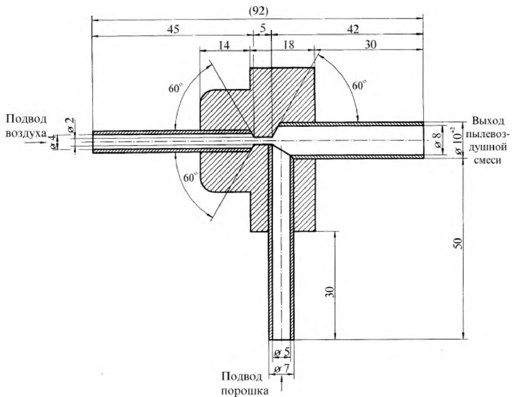
Рисунок 3 – Инжектор порошка
