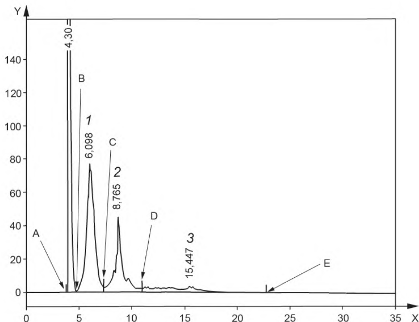
1 — моноароматические углеводороды; 2 — диароматические углеводороды; 3 — три-ароматические углеводороды; ось X — время, мин; ось Y — сигнал, мВ; A — начало пика неароматических углеводородов, t_a ; B — начало пика МАН, t_b ; C — впадина между МАН и ДАН t_c ; D — впадина между ДАН и Т+АН t_d ; E — конец площади интегрирования t_e
