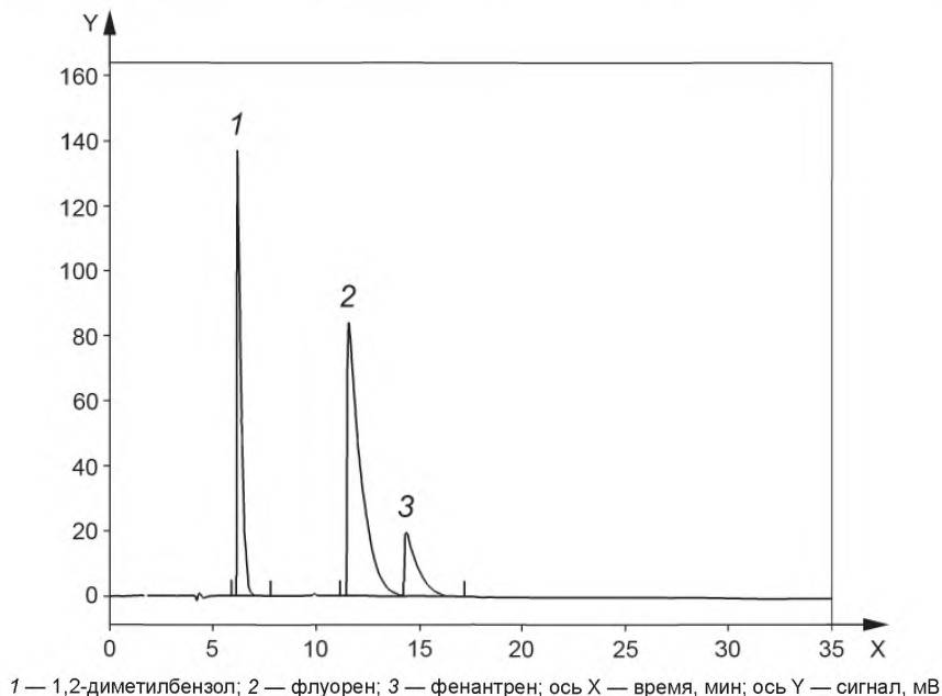
Рисунок 3 — Хроматограмма калибровочного стандартного раствора
